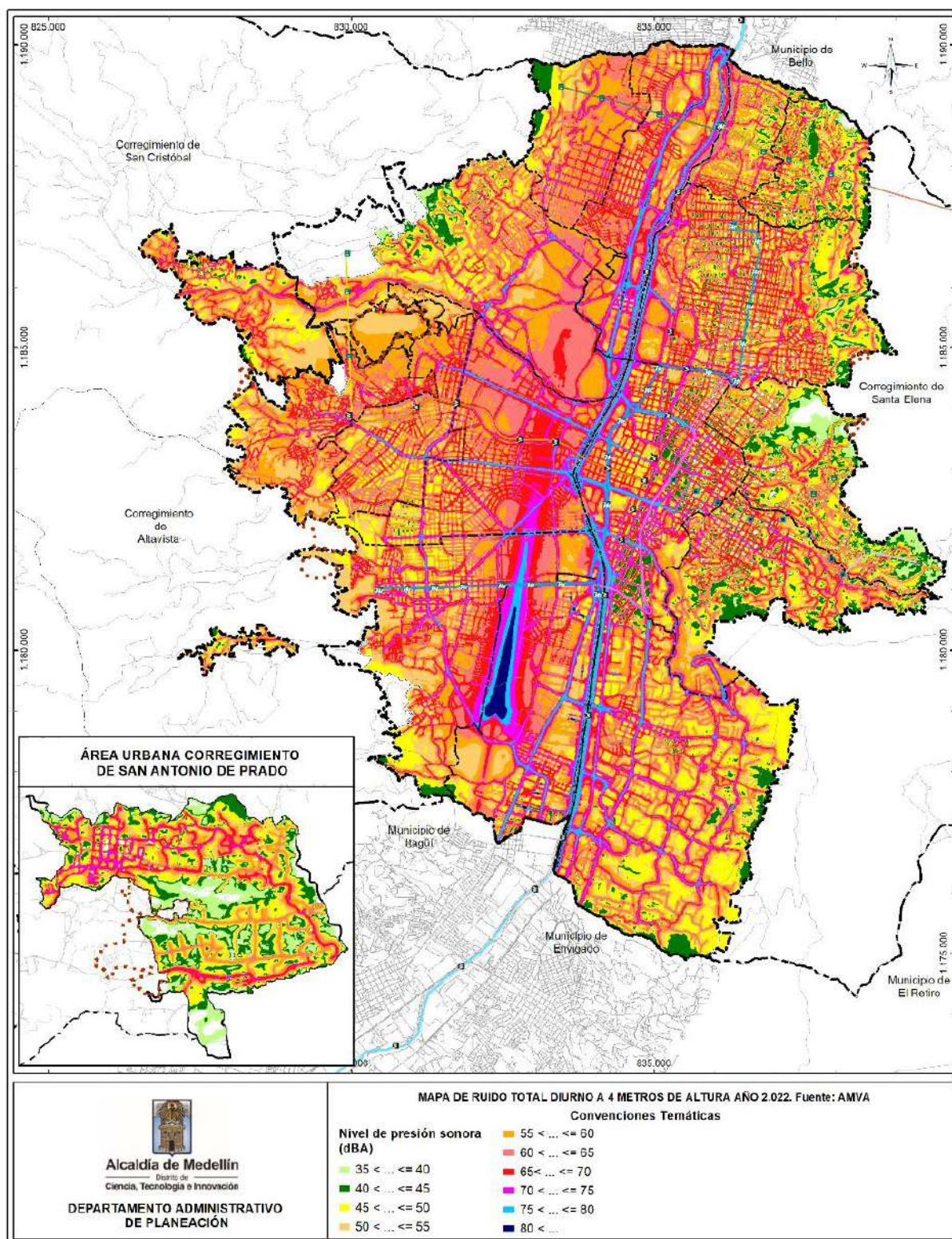
Figura 231. Mapa de Ruido Total Diurno a 4 metros de altura, año 2022
