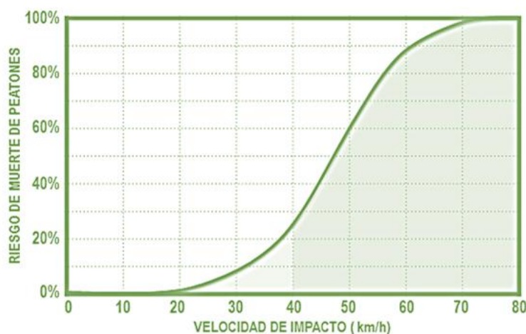
Figura 2-102 Relación Velocidad Riesgo de fatalidad peatonal en siniestro vial.
