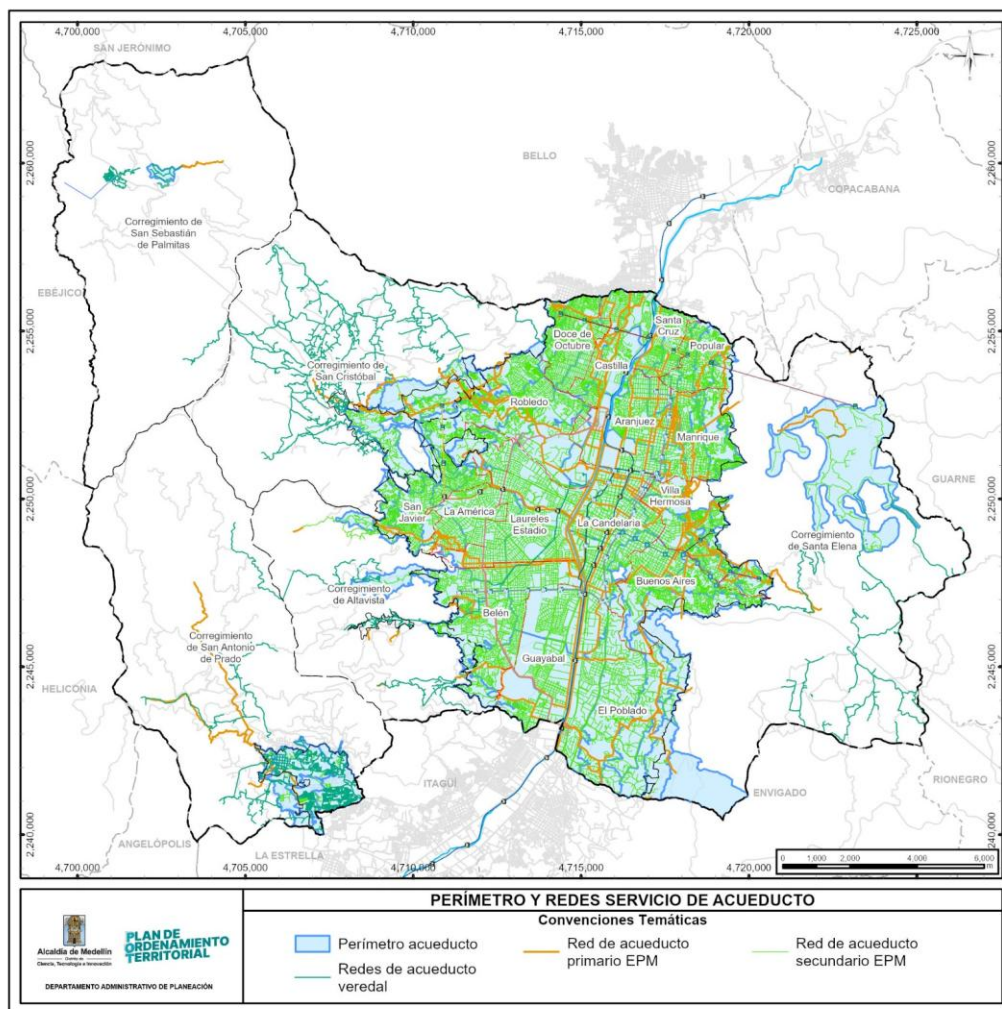
Figura 2-53. Redes de Acueducto y perímetro sanitario EPM.
