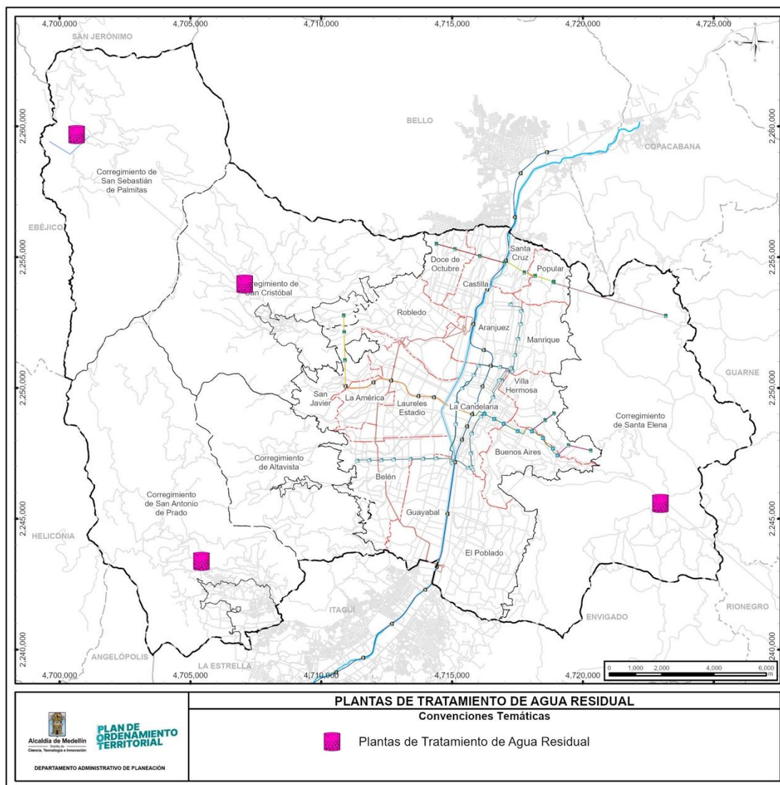
Figura 2-67. Localización de Plantas de tratamiento de agua residual.
