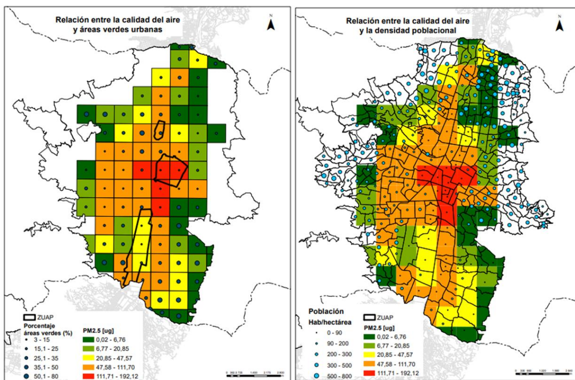
Figura 2-105. Producción de PM_{2.5} y población.
