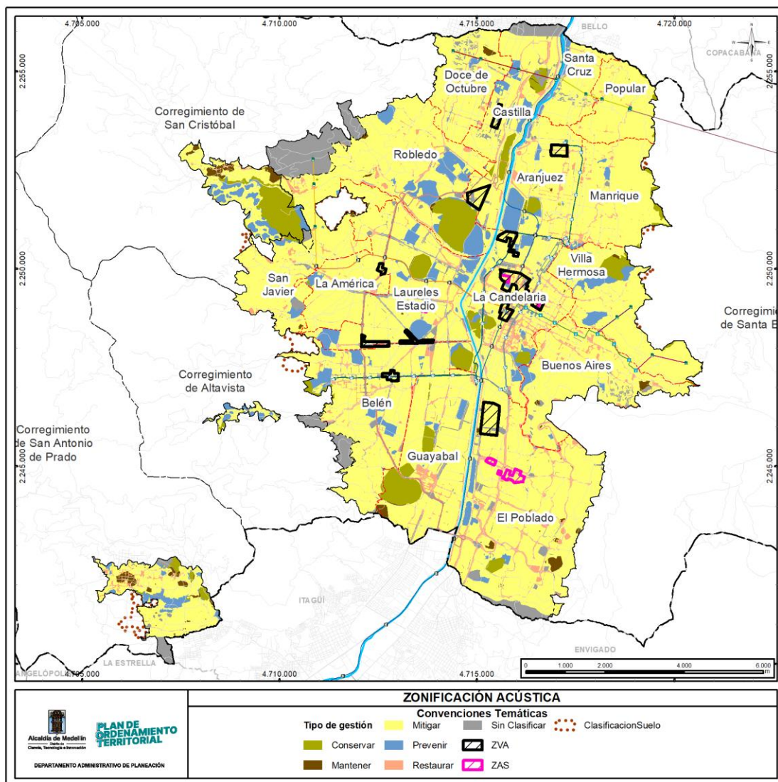
Figura 1-29. Zonificación acústica para el distrito de Medellín.
