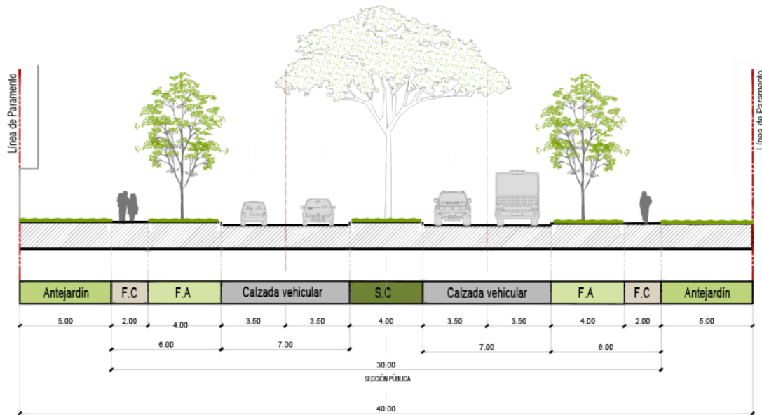
Figura 2-100. Sección mínima del POT para sistemas arteriales.
