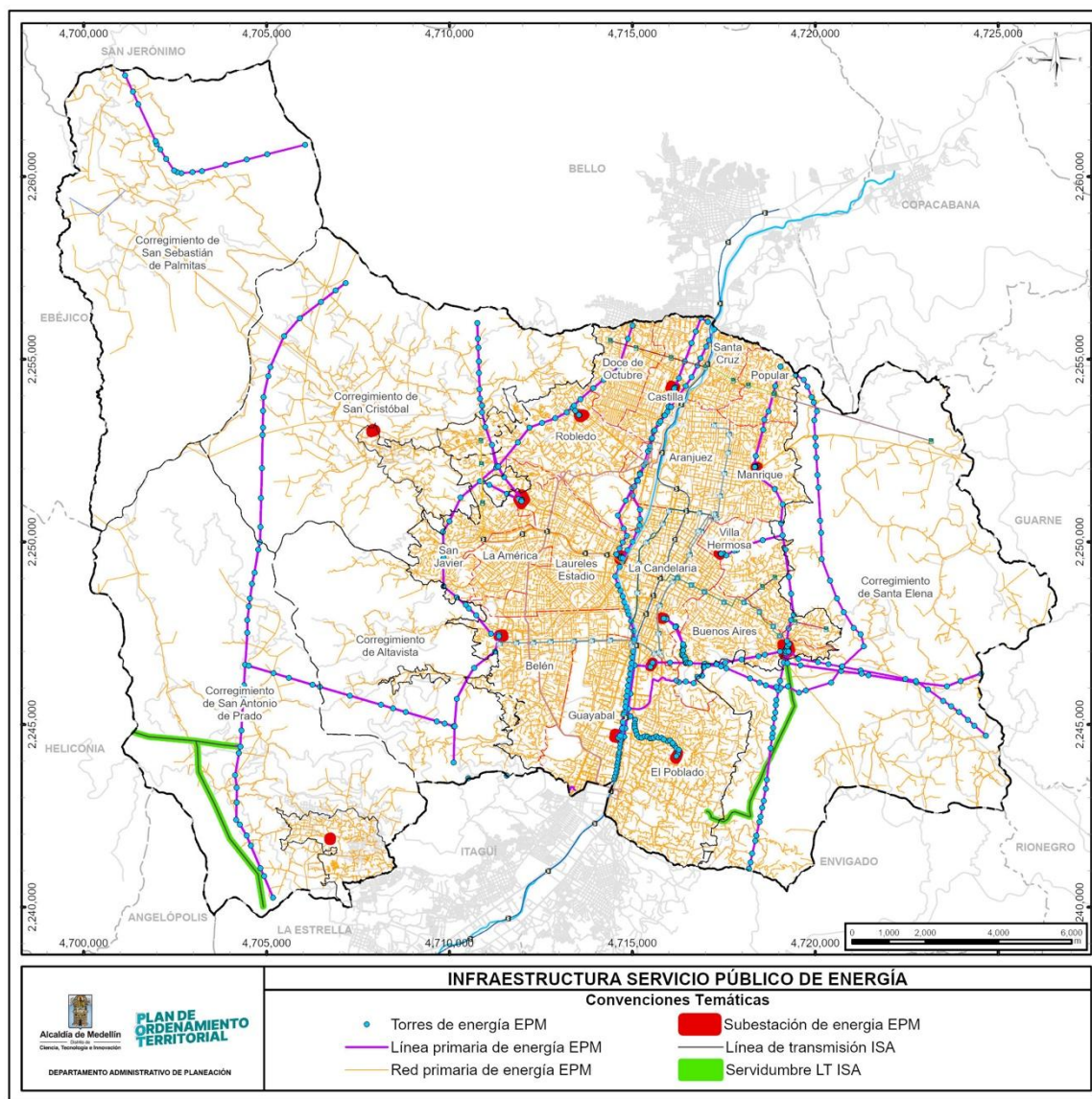
Figura 2-68. Redes y subestaciones de Energía.
