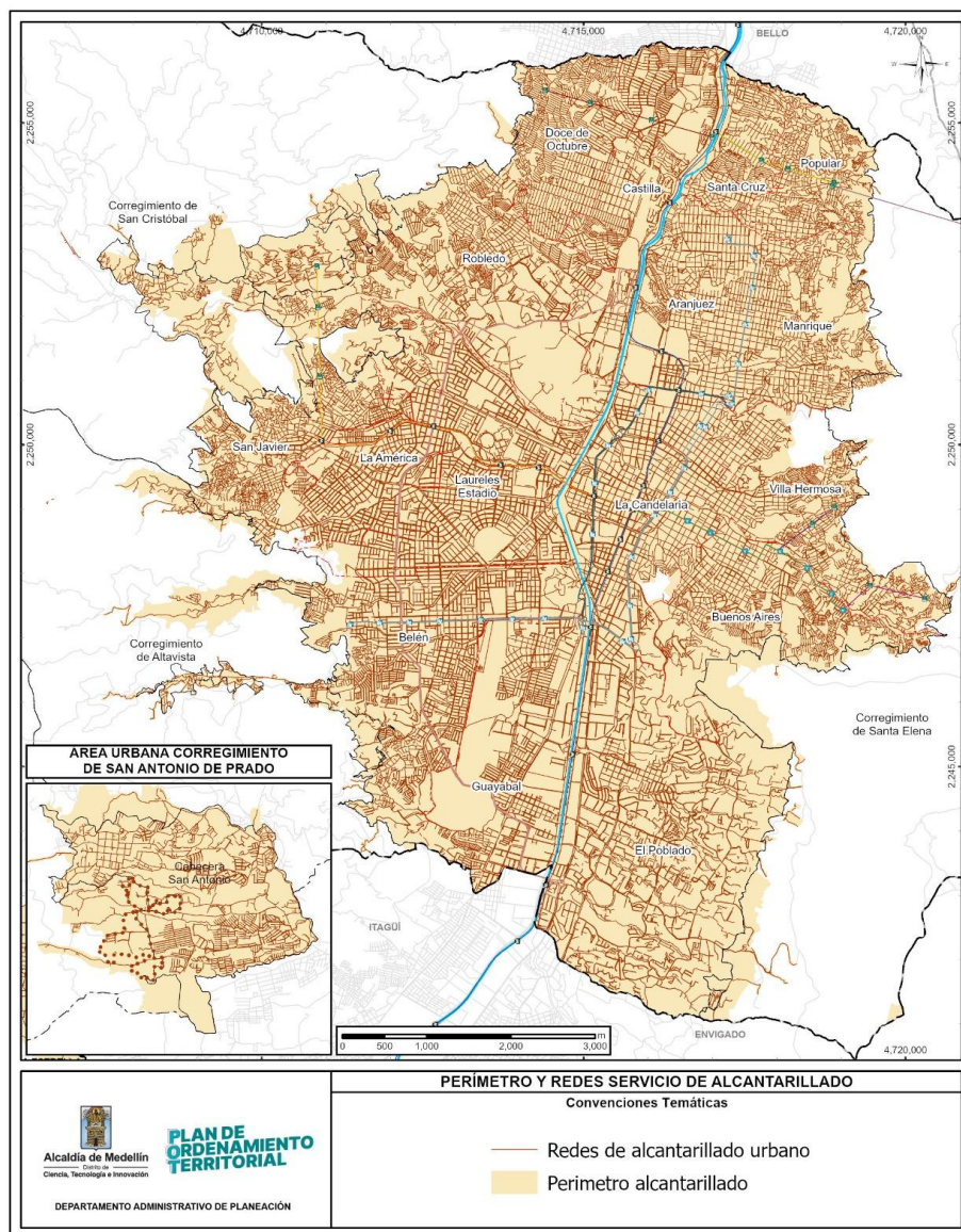
Figura 2-58. Redes de alcantarillado y perímetro Sanitario EPM.
