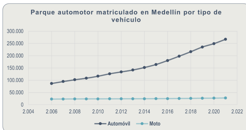
Figura 2-112. Parque automotor matriculado en Medellín por tipo de vehículo.
