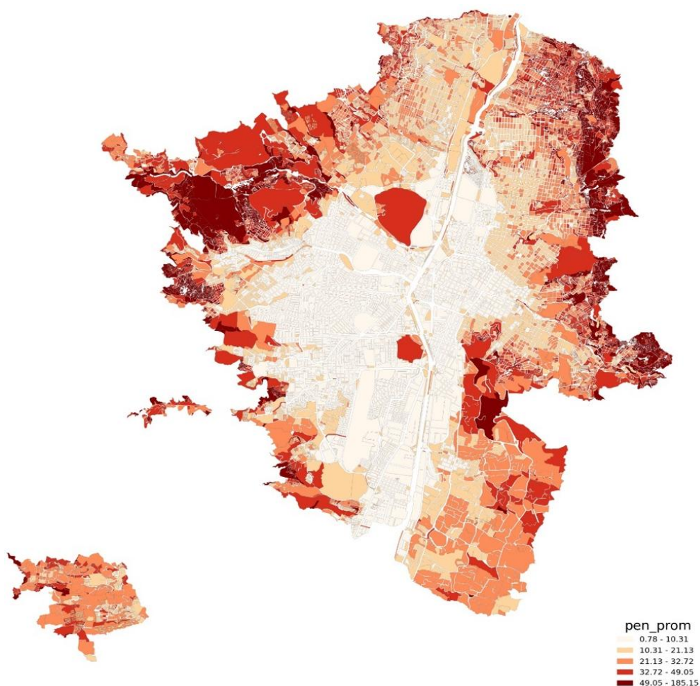
Figura 2-22. Pendiente promedio zona urbana.
