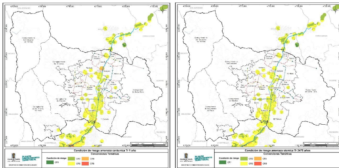
Figura 1-32. Condición de riesgo ante amenaza sísmica 475 años (izquierda) y 2475 años (derecha).
