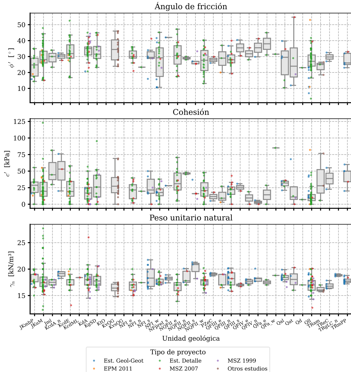
Ilustración 81. Distribución de los parámetros geomecánicos por unidad geológica y tipo de proyecto
