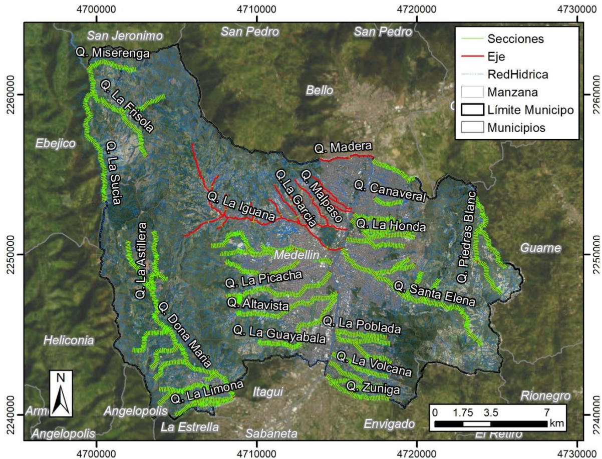
Ilustración 169. Secciones transversales en modelación hidráulica
