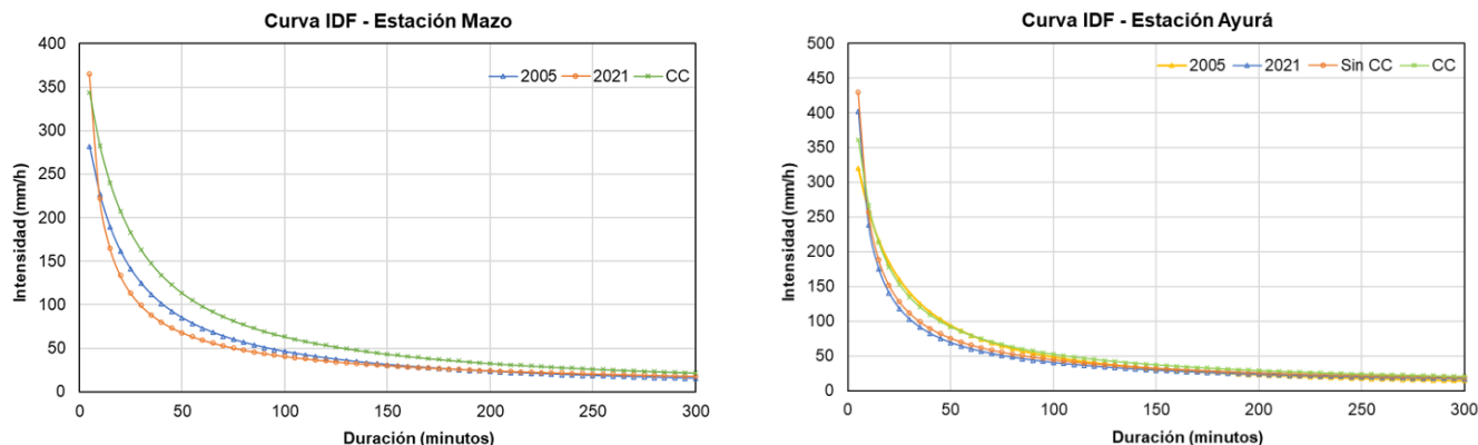
Ilustración 149. Comparación de diferentes estimaciones para las curvas IDF - T_R 100 años
