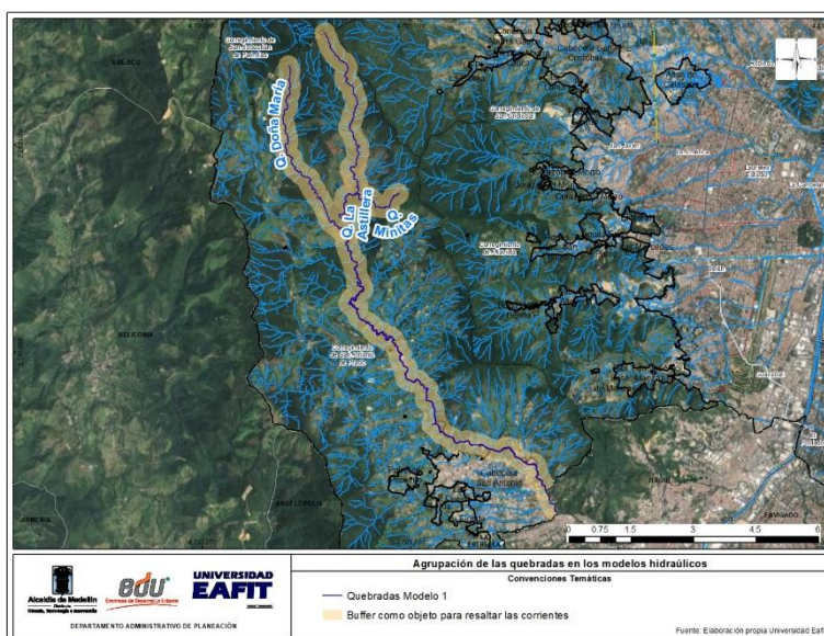
Ilustración 170 Fuentes hídricas incluidas en el modelo hidráulico 1
