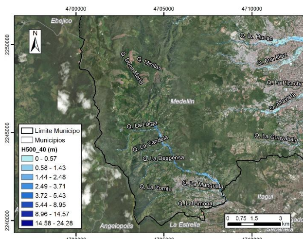
Profundidad TR500+40 Q. Doña María
