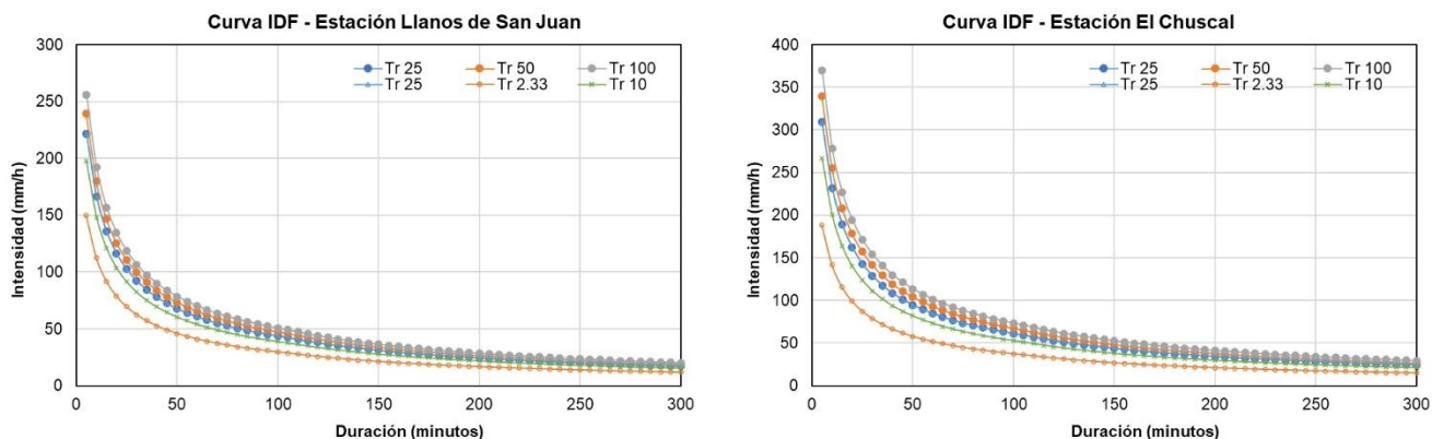
Ilustración 158. Curvas IDF para las estaciones Llanos de San Juan y El Chuscal
