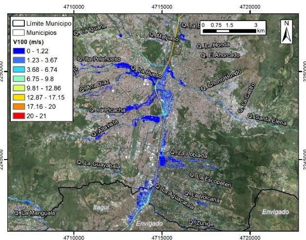
Velocidad TR100 Q. Santa Elena
