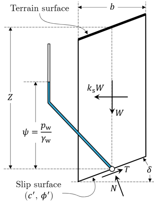
Ilustración 114. Mecanismo de talud infinito representativo de cada unidad de ladera para el análisis sísmico
