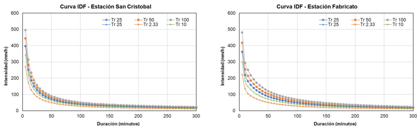
Ilustración 150. Curvas IDF para las estaciones San Cristóbal y Fabricato
