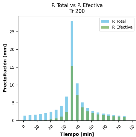
Ilustración 161. Aguacero de diseño en la quebrada Ana Díaz
