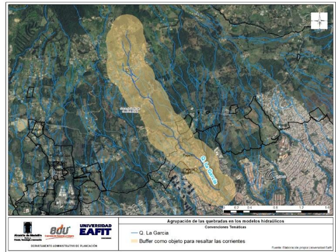
Ilustración 197. Fuentes hídricas incluidas en el modelo hidráulico La García
