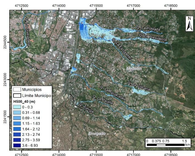
Profundidad TR500+40 Q. La Presidenta
