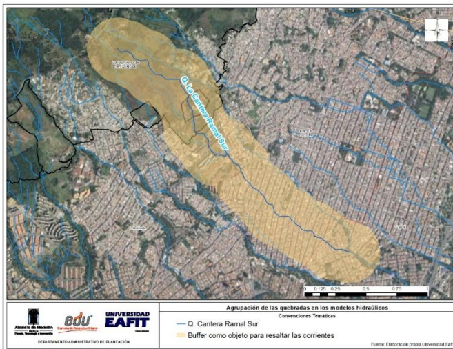
Ilustración 194. Fuentes hídricas incluidas en el modelo hidráulico La Cantera
