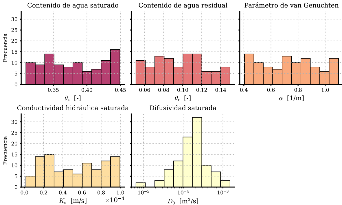
Ilustración 125. Histograma de las muestras aleatorias de los parámetros hidráulicos para el Distrito de Medellín
