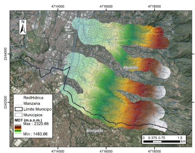
Geometría Q. La Presidenta
