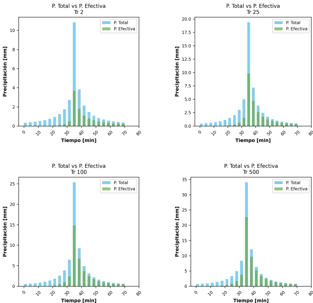
Ilustración 160. Aguacero de diseño en la quebrada La Presidenta
