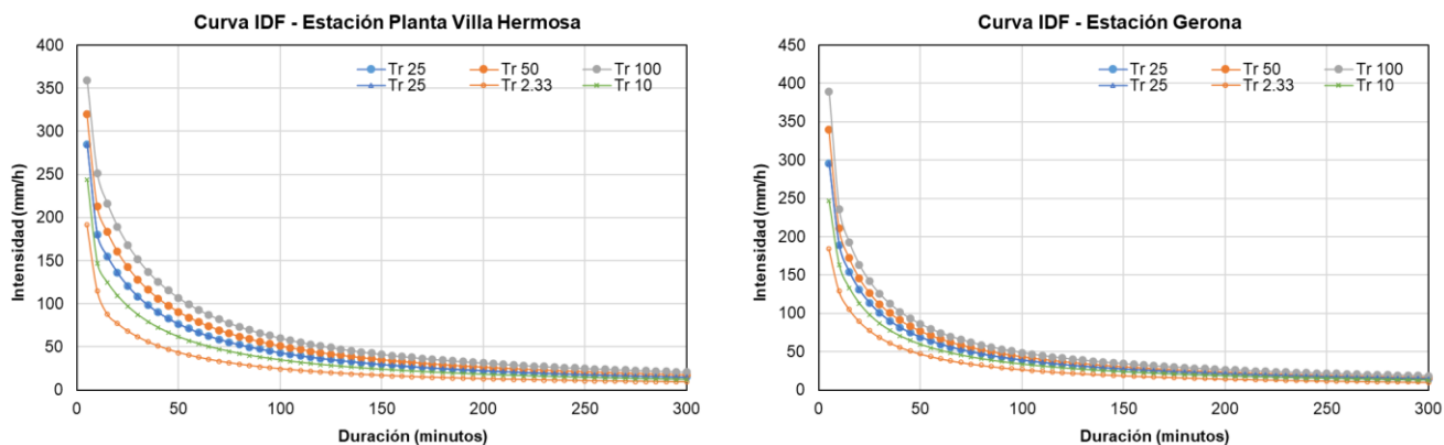
Ilustración 152. Curvas IDF para las estaciones Villa Hermosa y Gerona
