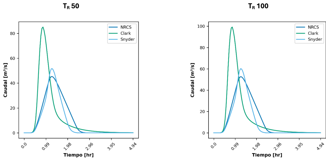
Ilustración 166. Hidrógrafa de respuesta de la quebrada La Aguacatala para Tr 50 años (izquierda) y 100 años (derecha).
