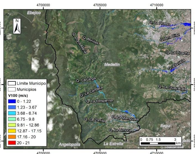
Velocidad TR100 Q. Doña María
