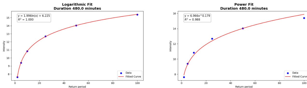
Ilustración 156. Ajuste logarítmico y potencial para un evento de duración de 480 minutos en la estación 2701037 (Fabricato) en el Escenario IDF 3
