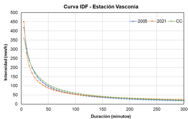
Ilustración 148. Comparación de diferentes estimaciones para las curvas IDF - T_R 100 años
