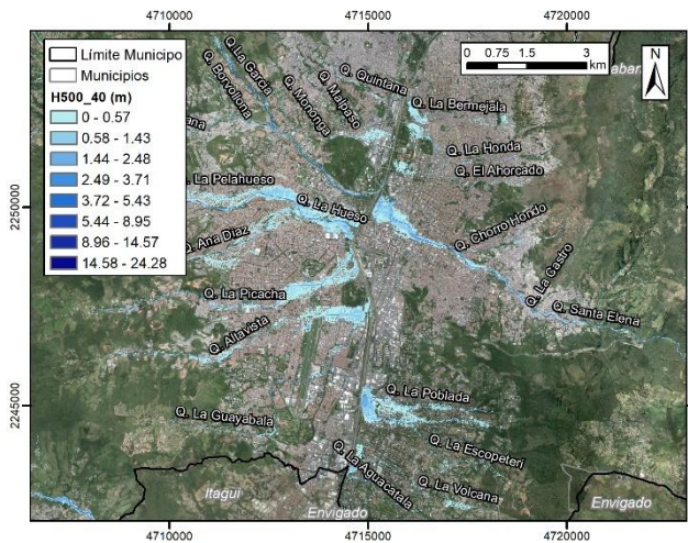
Profundidad TR500+40 Q. Santa Elena
