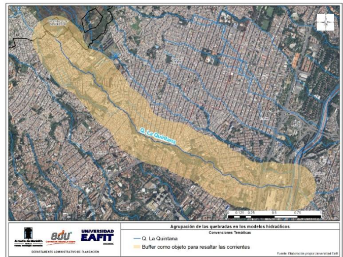
Ilustración 195. Fuentes hídricas incluidas en el modelo hidráulico La Quintana
