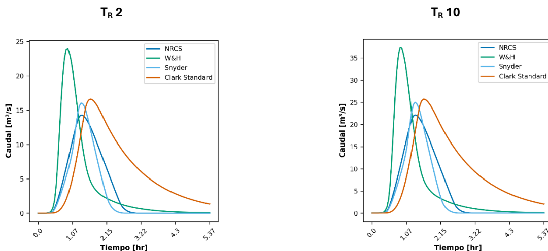
Ilustración 162. Hidrógrafa de respuesta de la quebrada Doña María para T_R 2 años (izquierda) y 10 años (derecha).
