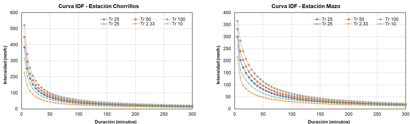
Ilustración 151. Curvas IDF para las estaciones Chorrillos y Mazo
