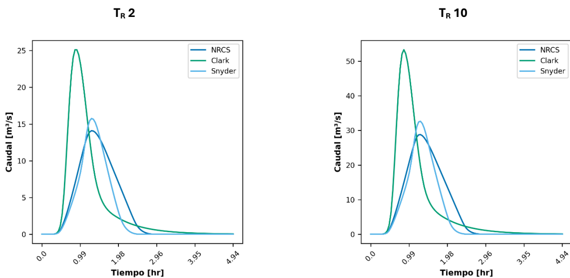
Ilustración 165. Hidrógrafa de respuesta de la quebrada La Aguacatala para T_R 2 años (izquierda) y 10 años (derecha).
