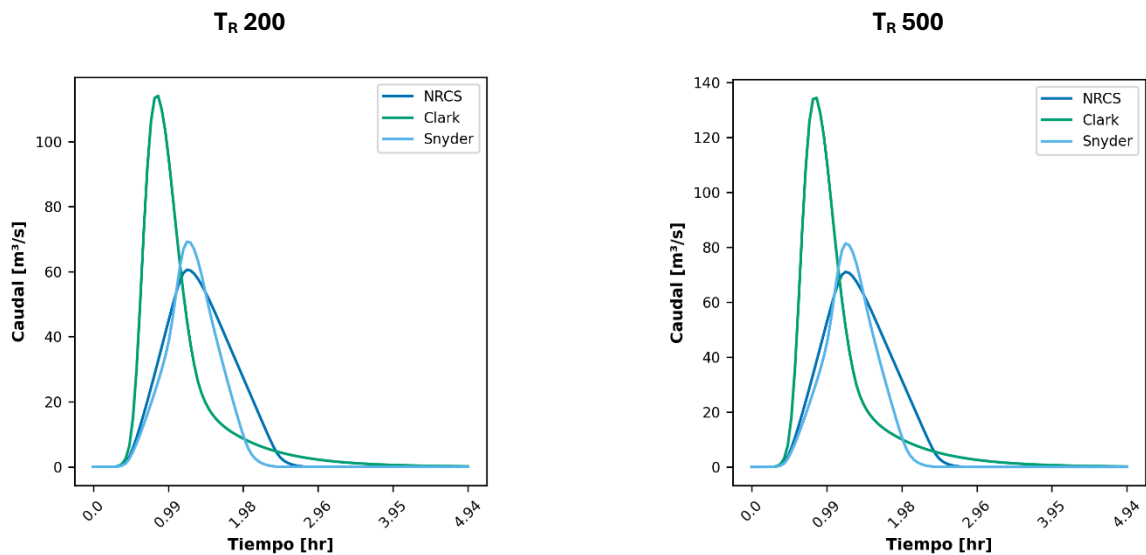
Ilustración 167. Hidrógrafa de respuesta de la quebrada La Aguacatala para Tr 200 años (izquierda) y 500 años (derecha).
