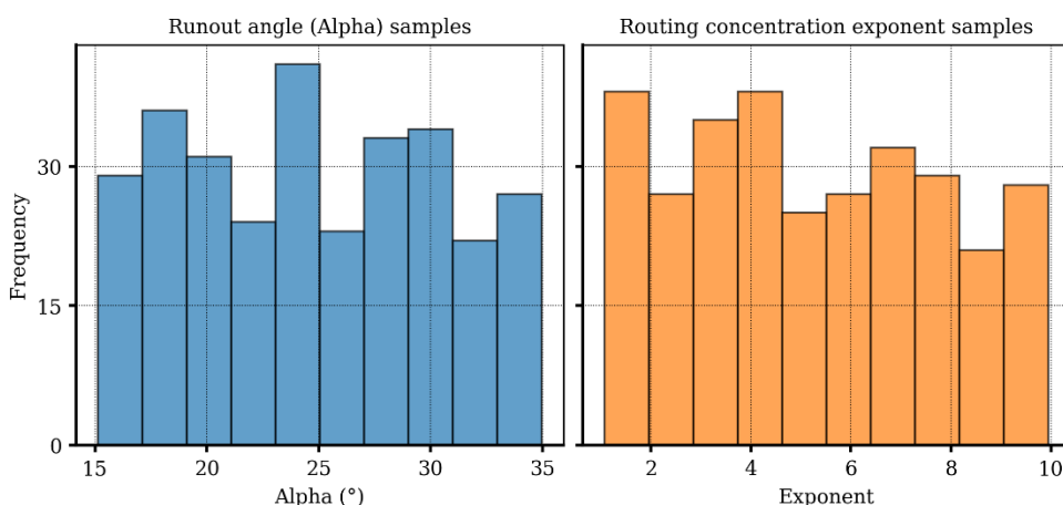
Ilustración 131. Histogramas de las muestras aleatorias para la modelación probabilista de propagación de deslizamientos
