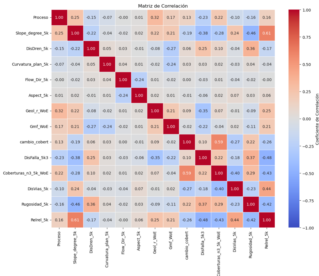
Ilustración 88. Ejemplo de matriz de correlación de Sperman evaluadas
