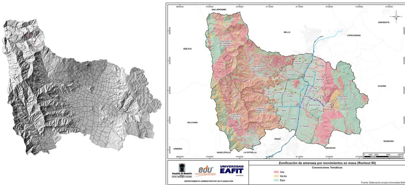
Ilustración 136. Áreas afectadas y zonificación de amenaza por índice de Probabilidad de Exposición a Propagación mayor a 50%.
