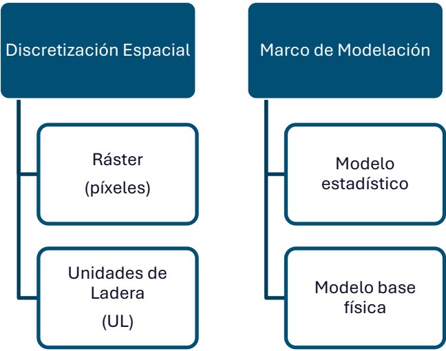
Ilustración 86. Esquema de la discretización espacial y el marco de modelación desarrollados para el Distrito de Medellín
