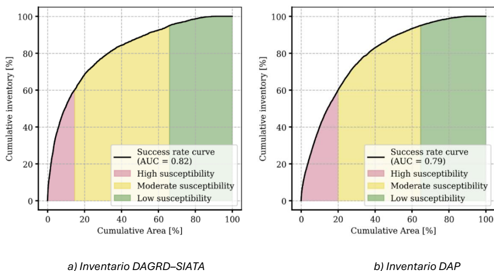
Ilustración 101. Curva de éxito, área bajo la curva y delimitación de umbrales para la zonificación por píxeles
