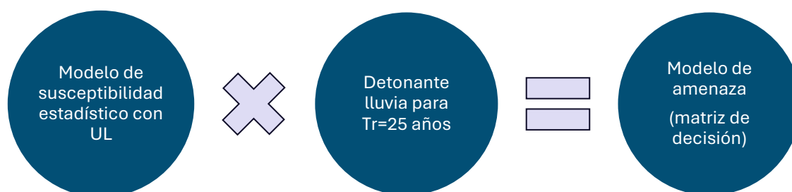
Ilustración 117. Esquema de estimación del modelo de amenaza por movimientos en masa para el Distrito de Medellín
