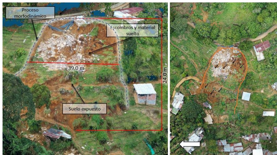
Ilustración 69 Deslizamiento en vereda Piedras Blancas - Matasano
