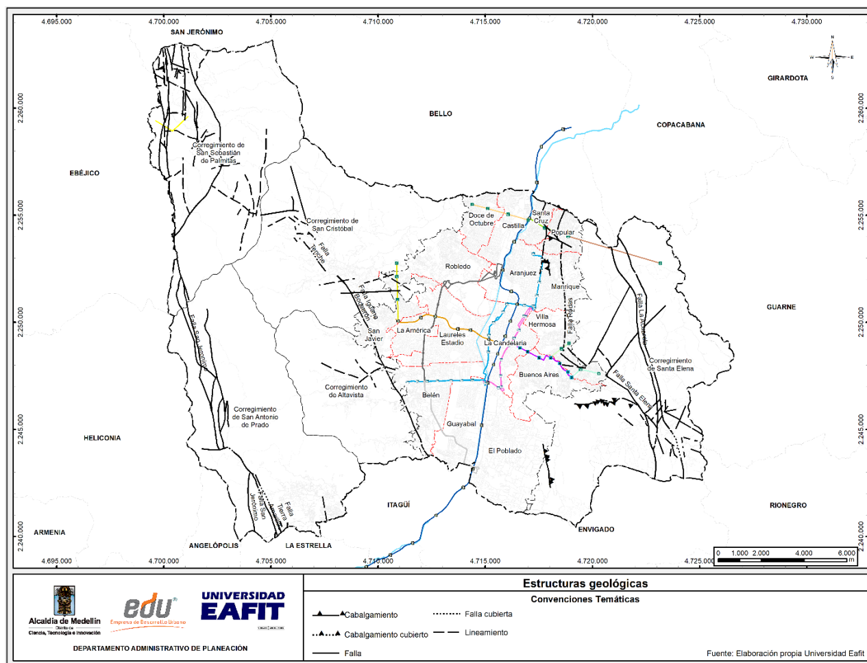
Ilustración 25 Estructuras geológicas en el distrito de Medellín
