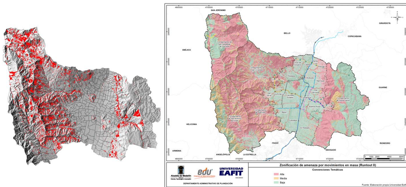
Ilustración 133. Áreas afectadas y zonificación de amenaza por índice de Probabilidad de Exposición a Propagación mayor a 0%.
