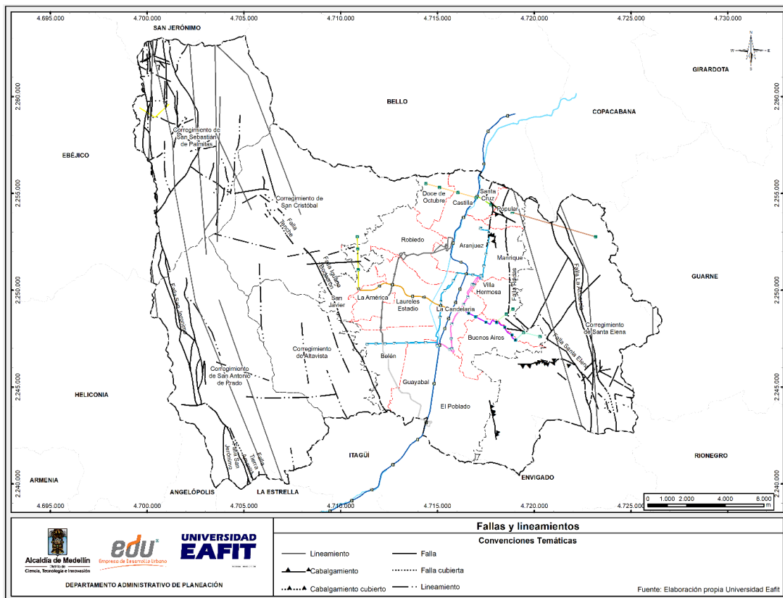
Ilustración 7 Fallas y lineamientos en el distrito de Medellín
