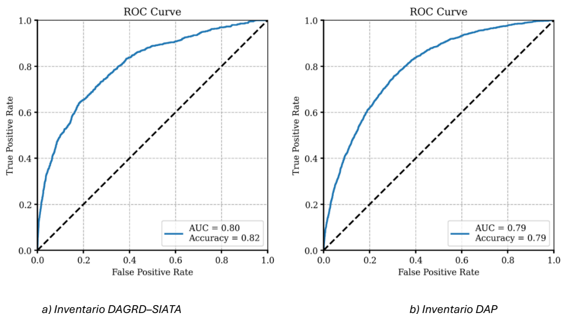
Ilustración 105. Curva ROC del modelo de red neuronal para UL
