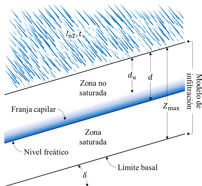
Ilustración 3. Esquema de las componentes del modelo TRIGRS
