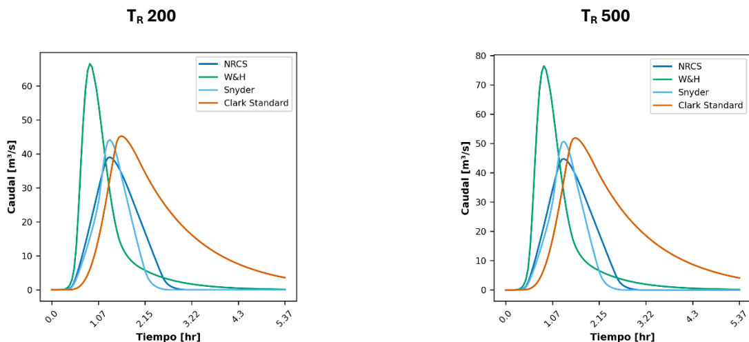
Ilustración 164. Hidrógrafa de respuesta de la quebrada Doña María para T_R 200 años (izquierda) y 500 años (derecha).
