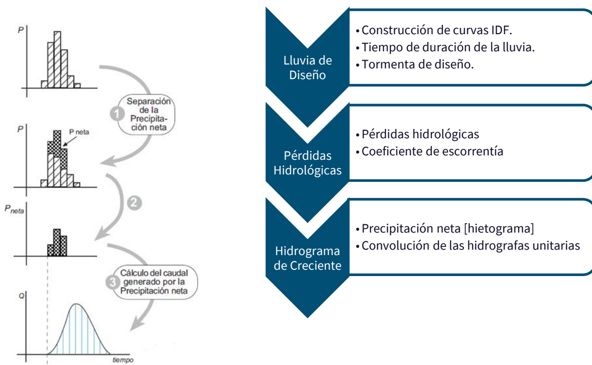
Ilustración 145. Esquematzación del proceso de estimación de caudales máximos
