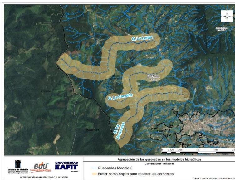
Ilustración 171. Fuentes hídricas incluidas en el modelo hidráulico 2
