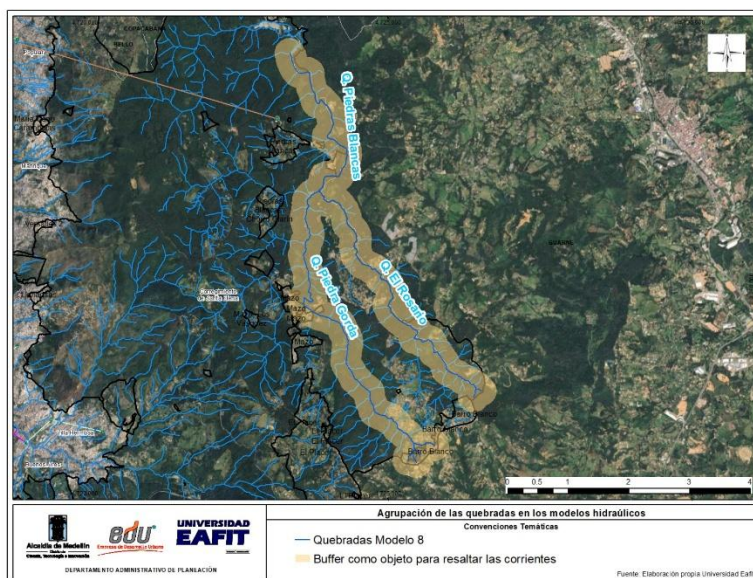
Ilustración 177. Fuentes hídricas incluidas en el modelo hidráulico 8
