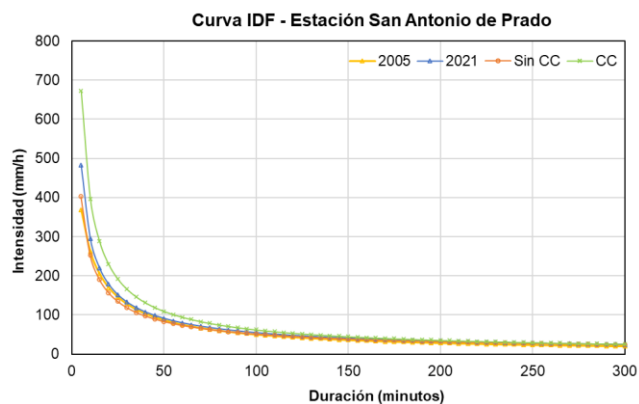
Ilustración 147. Comparación de diferentes estimaciones para las curvas IDF - T_R 100 años
