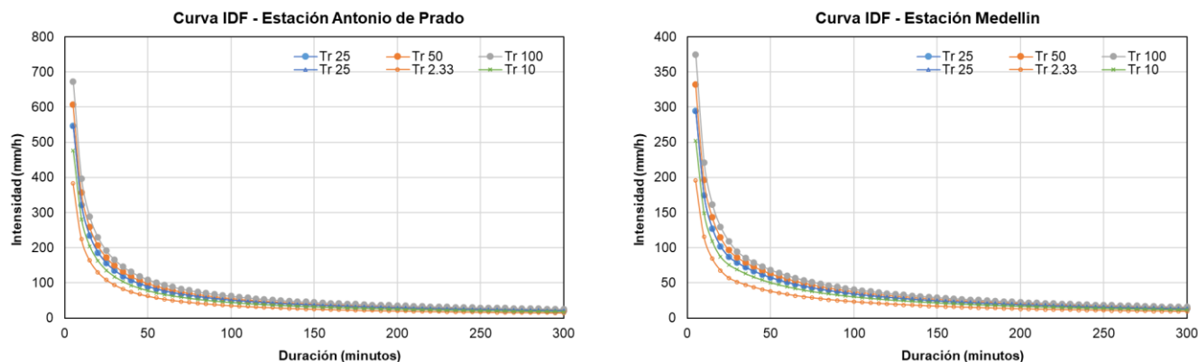
Ilustración 154. Curvas IDF para las estaciones San Antonio de Prado y Medellín
