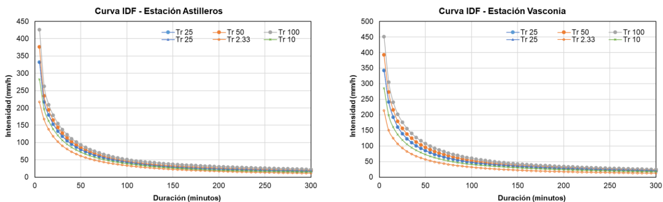
Ilustración 153. Curvas IDF para las estaciones Astillero y Vasconia
