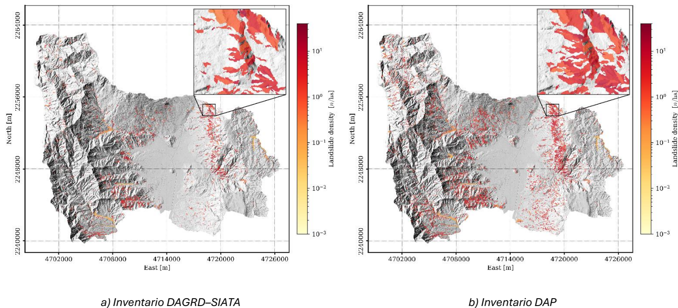
Ilustración 85. Densidad de deslizamientos por área en cada UL en el Distrito de Medellín
