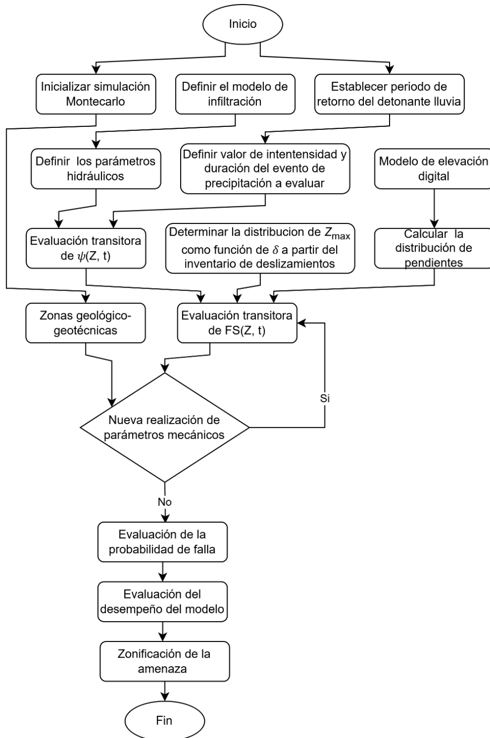
Ilustración 288. Metodología para la evaluación de la amenaza por movimientos en masa a partir de la probabilidad espacial de falla
