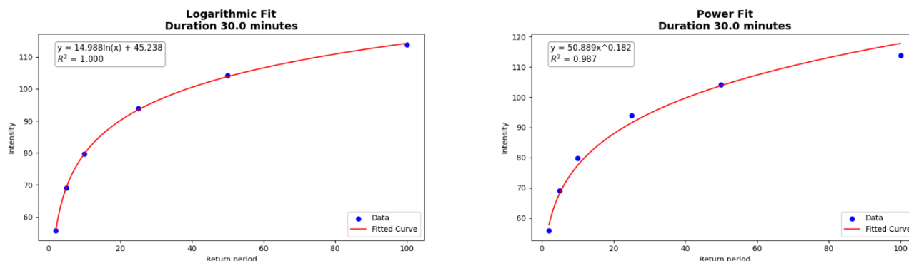
Ilustración 157. Ajuste logarítmico y potencial para un evento de duración de 30 minutos en la estación 2701046 (San Cristóbal) – En el Escenario IDF 1
