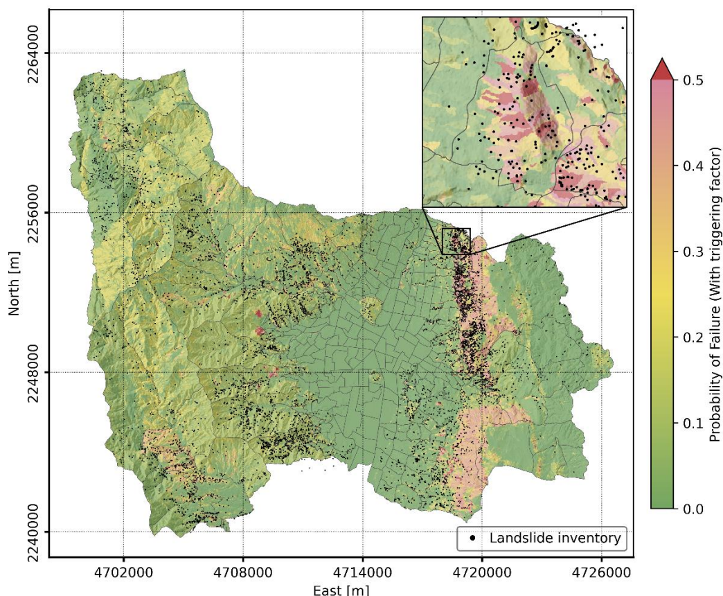
Ilustración 129. Distribución espacial de la probabilidad de falla para el detonante lluvia con T_r de 25 años en el Distrito de Medellín
