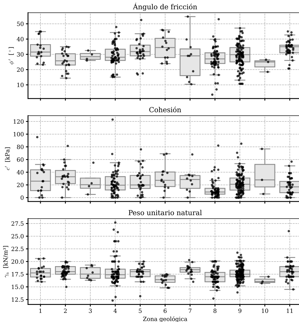
Ilustración 82. Distribución de los parámetros geomecánicos por zona geológica
