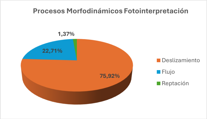
Ilustración 57. Eventos fotointerpretación
