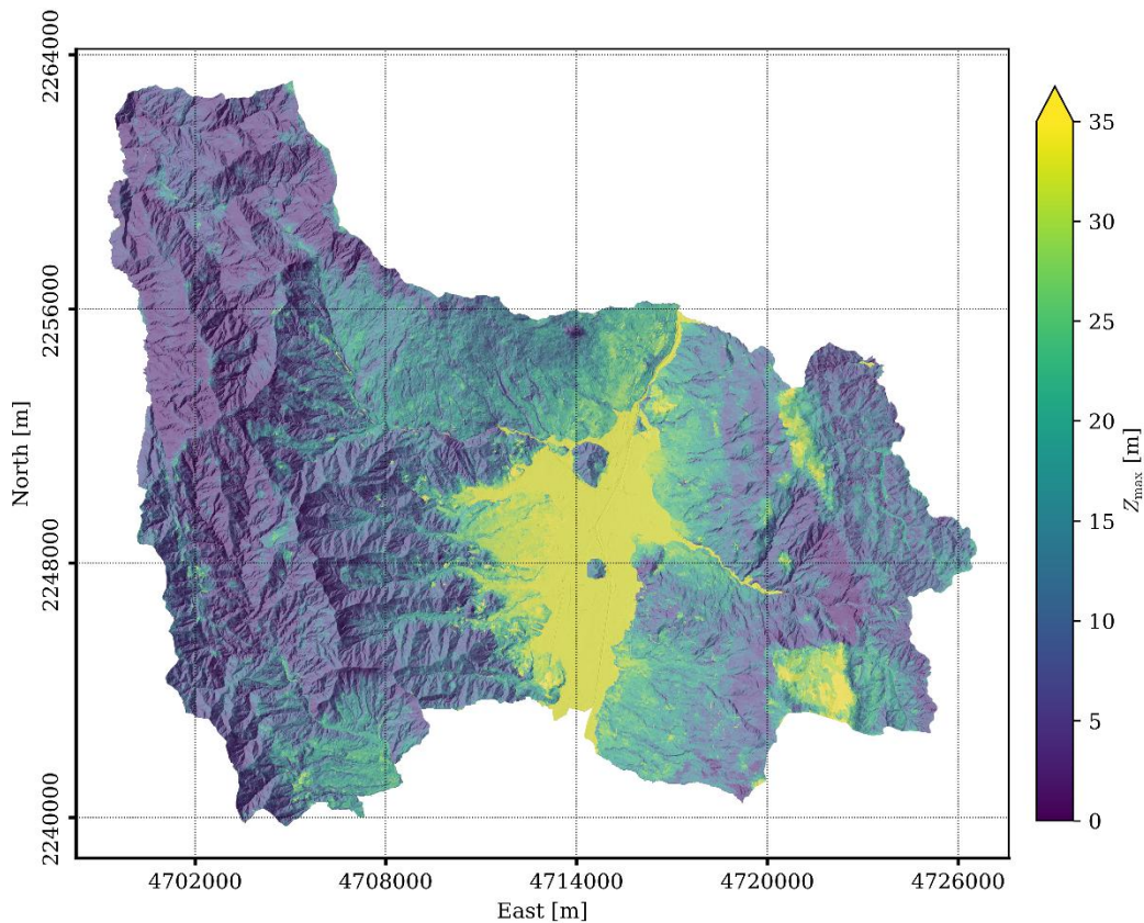
Ilustración 108. Distribución espacial de Z_{\max} para un modelo exponencial empírico en el Distrito de Medellín
