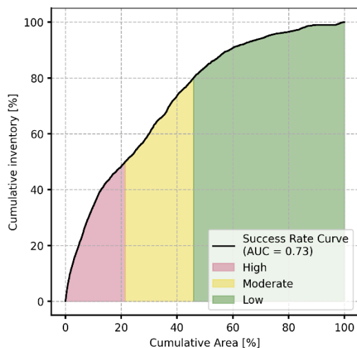
Ilustración 127. Curva de éxito, área bajo la curva y delimitación de umbrales para la zonificación
