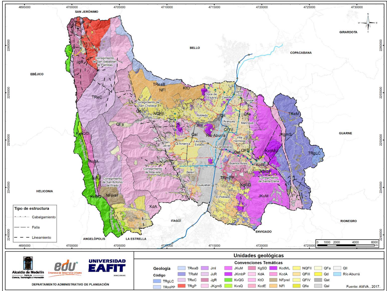
Ilustración 9. Mapa de unidades geológicas locales del Distrito de Medellín
