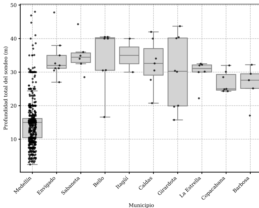
Ilustración 80. Distribución de profundidades de los sondeos de exploración geotécnica para el Distrito de Medellín y los municipios del Área Metropolitana
