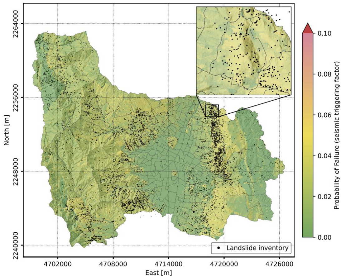
Ilustración 115. Probabilidad de falla sísmica a una escala temporal equivalente de T_r = 25 años
