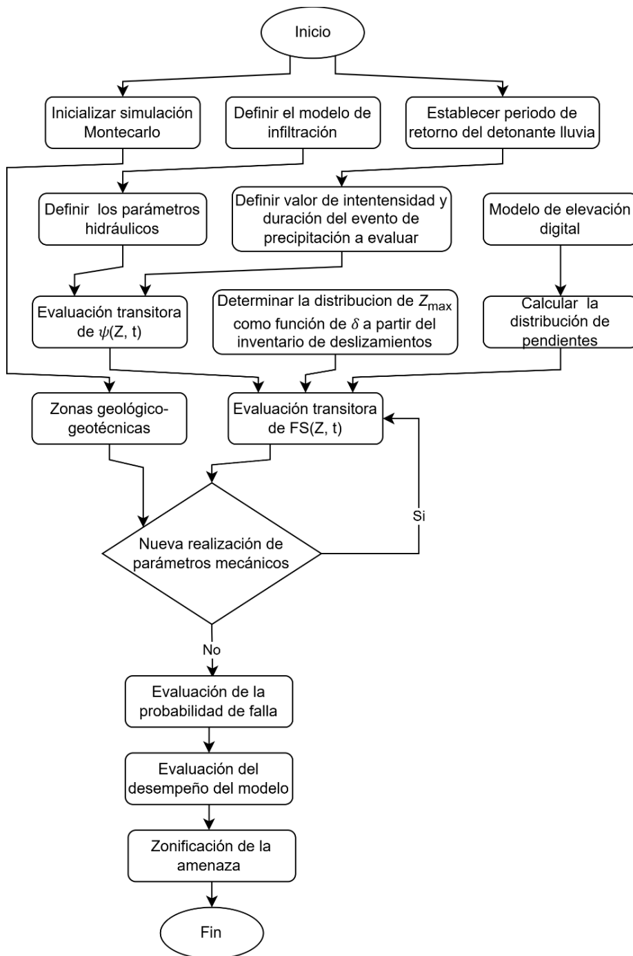
Ilustración 4. Metodología para la evaluación de la amenaza por movimientos en masa a partir de la probabilidad espacial de falla
