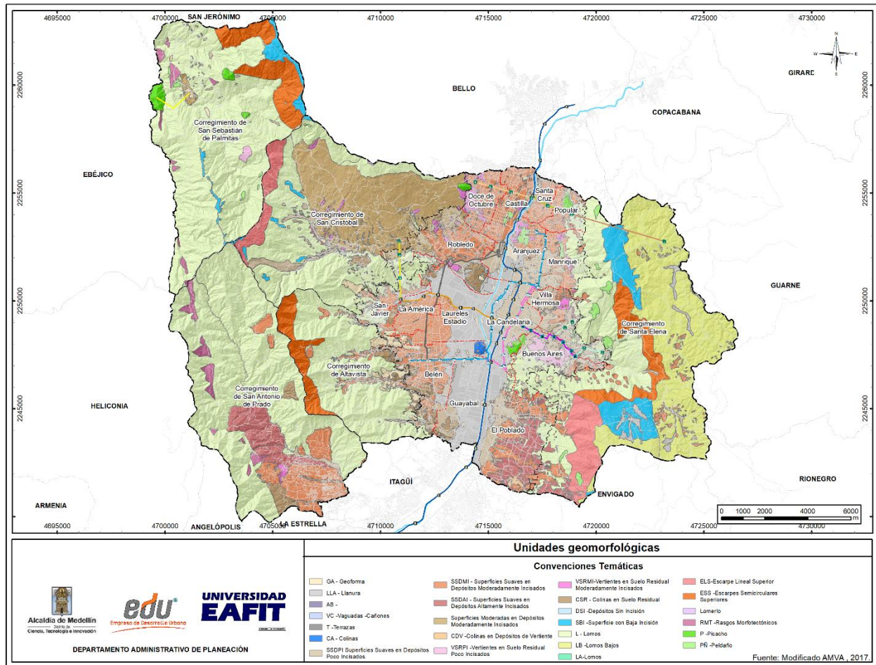
Ilustración 26. Mapa de unidades geomorfológicas del Distrito de Medellín
