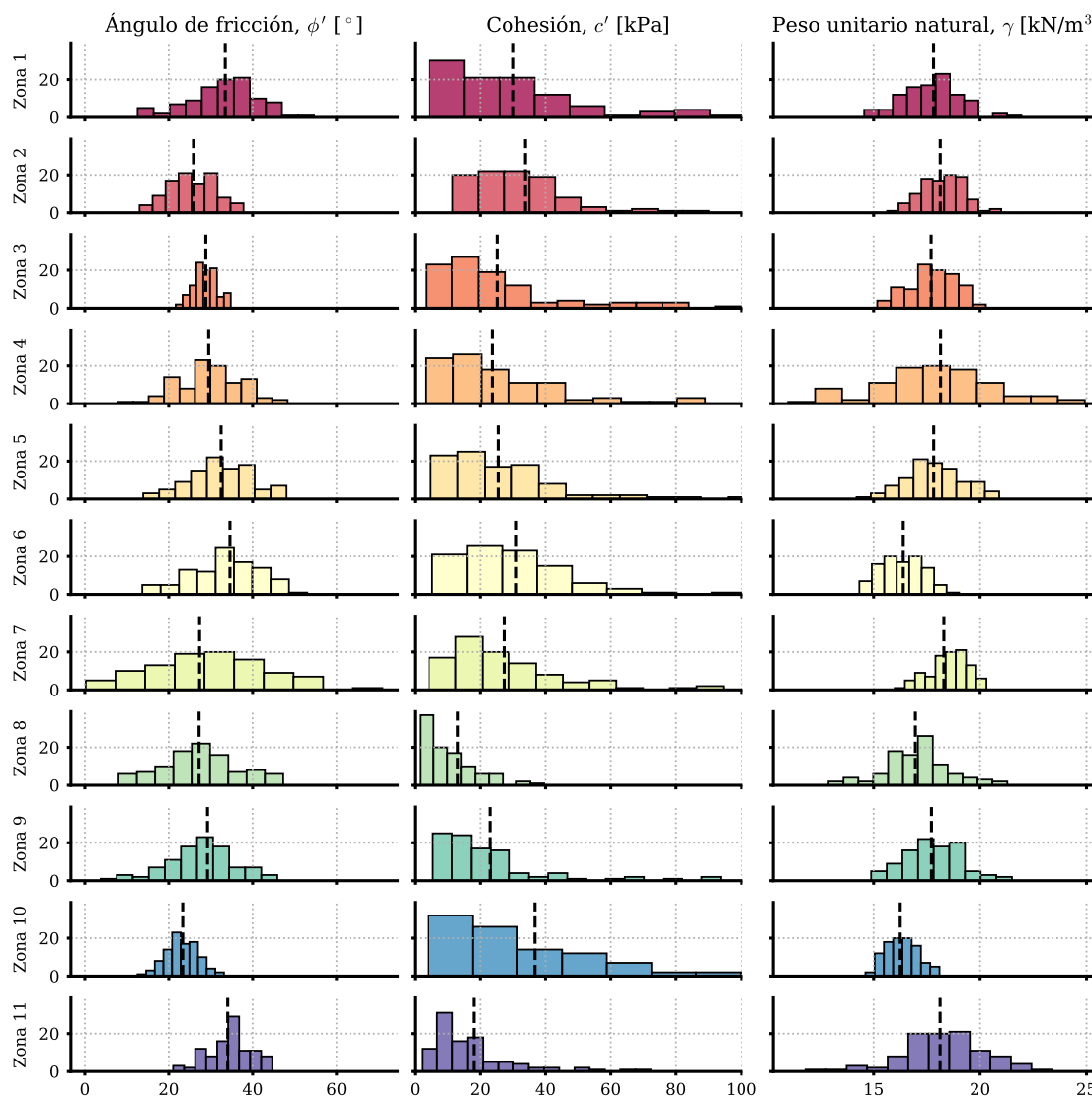
Ilustración 124. Histograma de las muestras aleatorias de los parámetros geomecánicos para cada zona geológica
