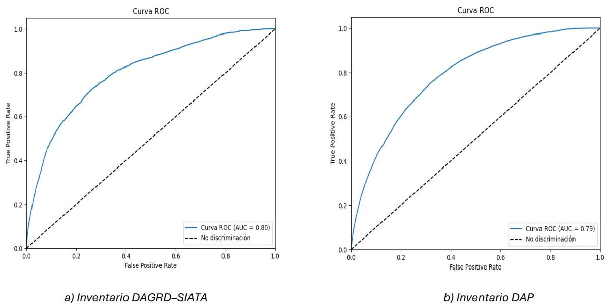
Ilustración 91. Curva ROC del modelo de peso de la evidencia
