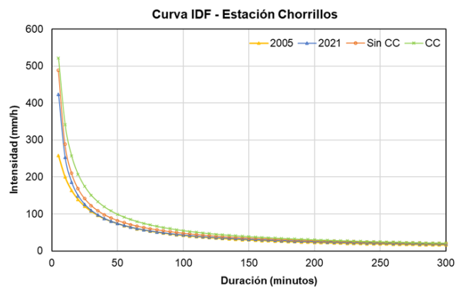
Ilustración 146. Comparación de diferentes estimaciones para las curvas IDF - T_R 100 años
