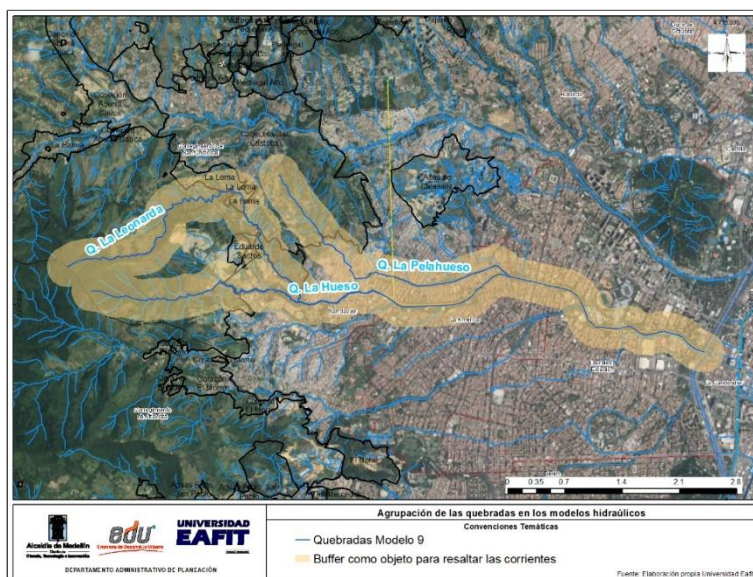
Ilustración 178. Fuentes hídricas incluidas en el modelo hidráulico 9
