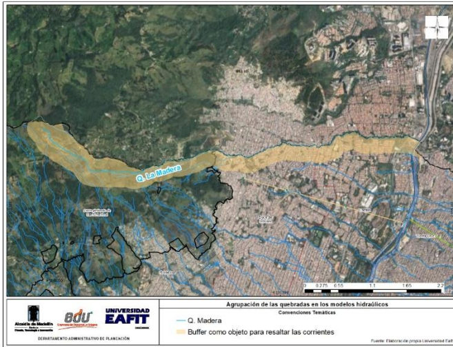
Ilustración 192. Fuentes hídricas incluidas en el modelo hidráulico La Madera
