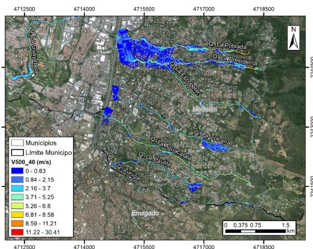
Velocidad TR500+40 Q. La Presidenta
