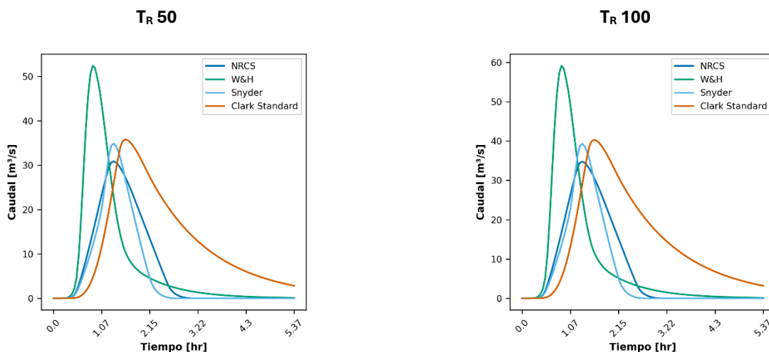
Ilustración 163. Hidrógrafa de respuesta de la quebrada Doña María para T_R 50 años (izquierda) y 100 años (derecha).
