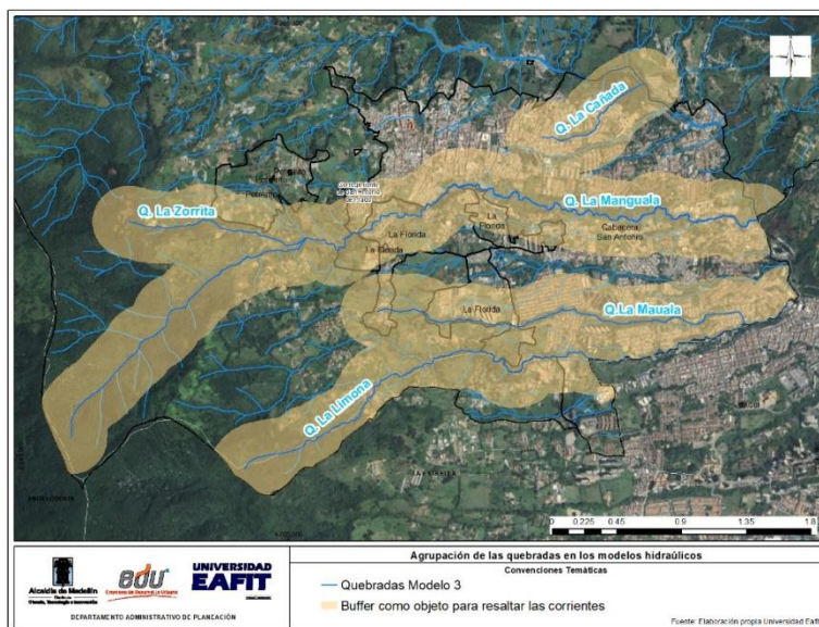
Ilustración 172. Fuentes hídricas incluidas en el modelo hidráulico 3
