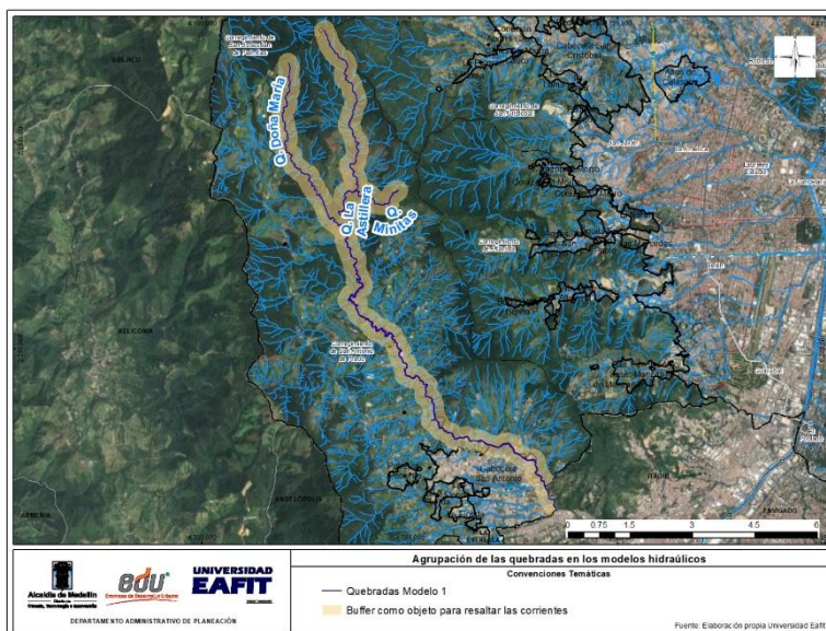
Ilustración 170 Fuentes hídricas incluidas en el modelo hidráulico 1
