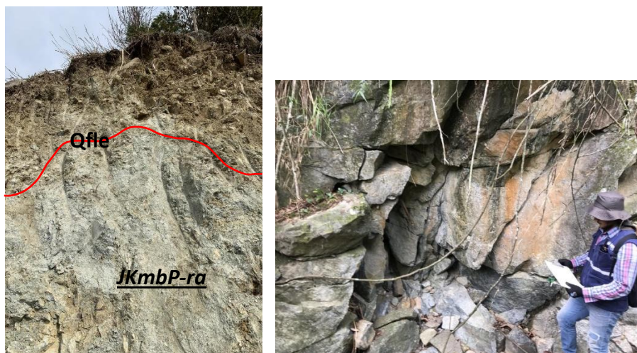
Ilustración 14. Nivel IIA y roca fracturada reportada sobre la margen derecha de la quebrada Malpaso
