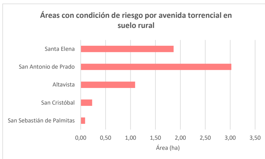
Ilustración 247. Áreas con condición de riesgo por avenidas torrenciales en el suelo de rural del Distrito de Medellín
