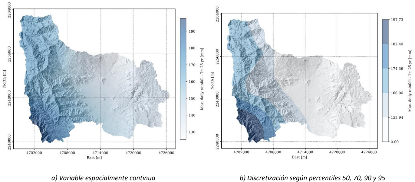
Ilustración 113. Distribución espacial de la lluvia diaria máxima estimada para un T_r de 25 años en el Distrito de Medellín
