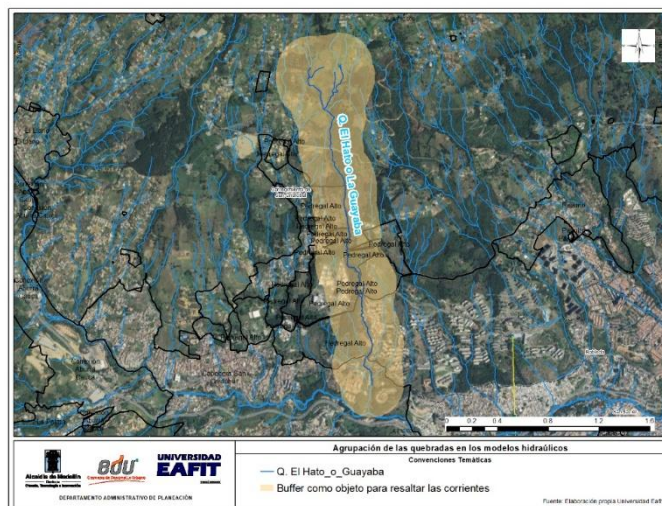
Ilustración 189. Fuentes hídricas incluidas en el modelo hidráulico El Hato
