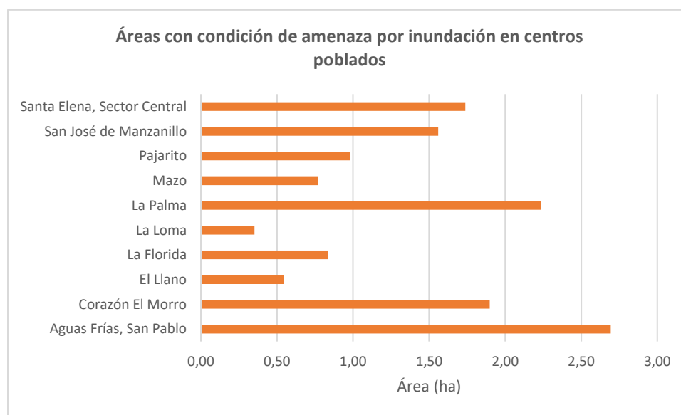
Ilustración 260. Áreas con condición de amenaza por inundaciones en los centros poblados del Distrito de Medellín
