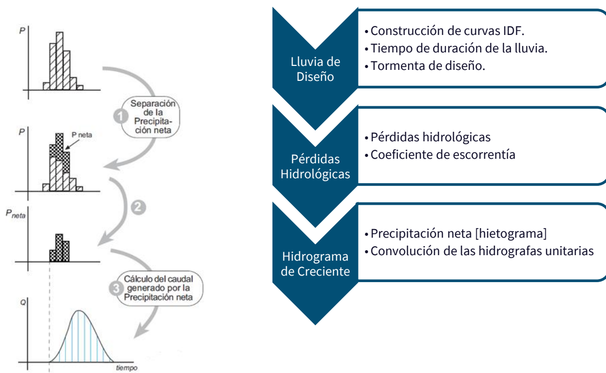
Ilustración 145. Esquemización del proceso de estimación de caudales máximos
