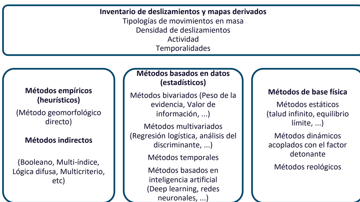
Ilustración 1. Clasificación de los métodos para la evaluación de la amenaza por movimientos en masa
