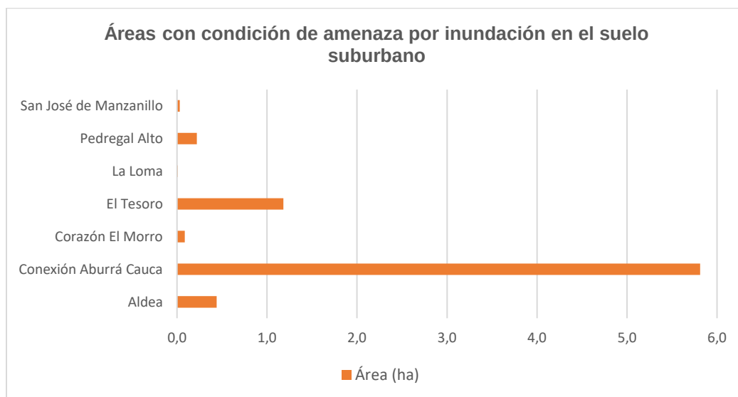
Ilustración 254. Áreas con condición de amenaza por avenidas torrenciales del suelo suburbano del Distrito de Medellín
