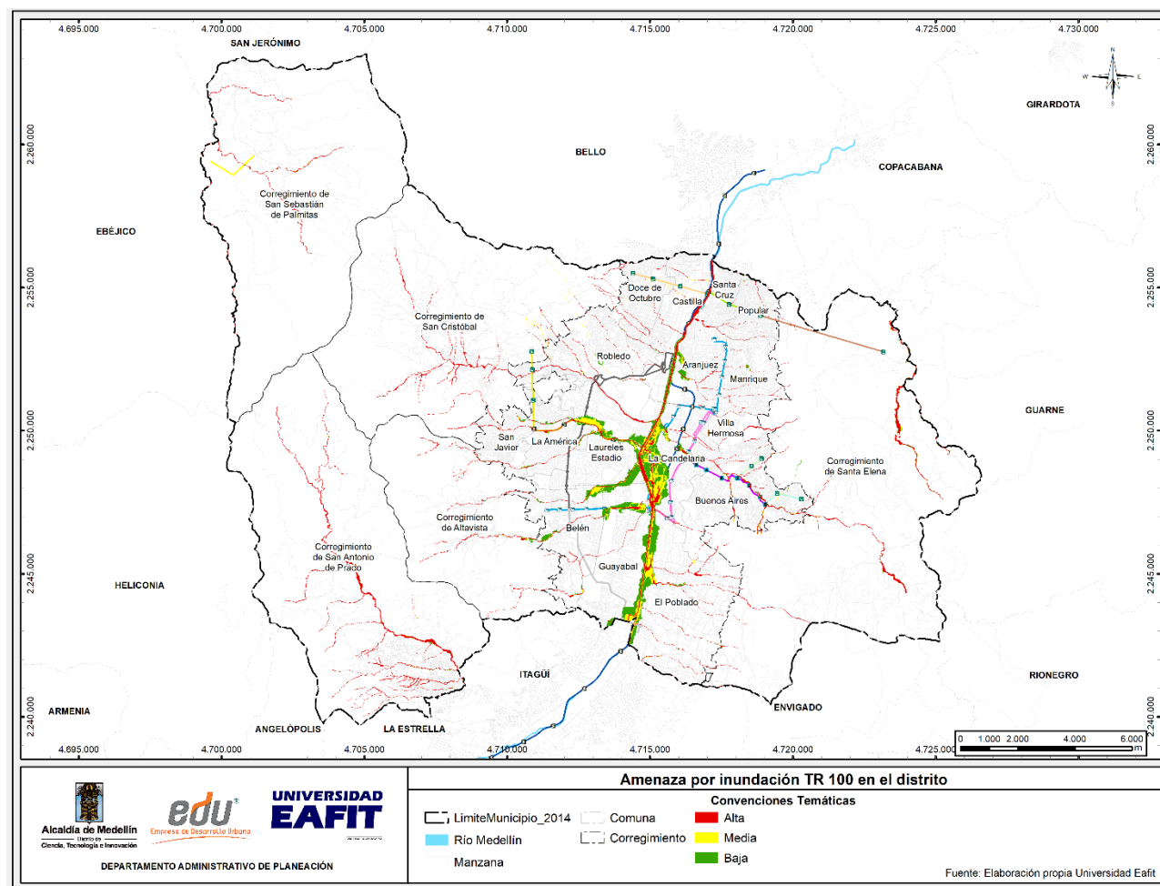
Ilustración 217. Zonificación de la amenaza por inundación en el Distrito de Medellín
