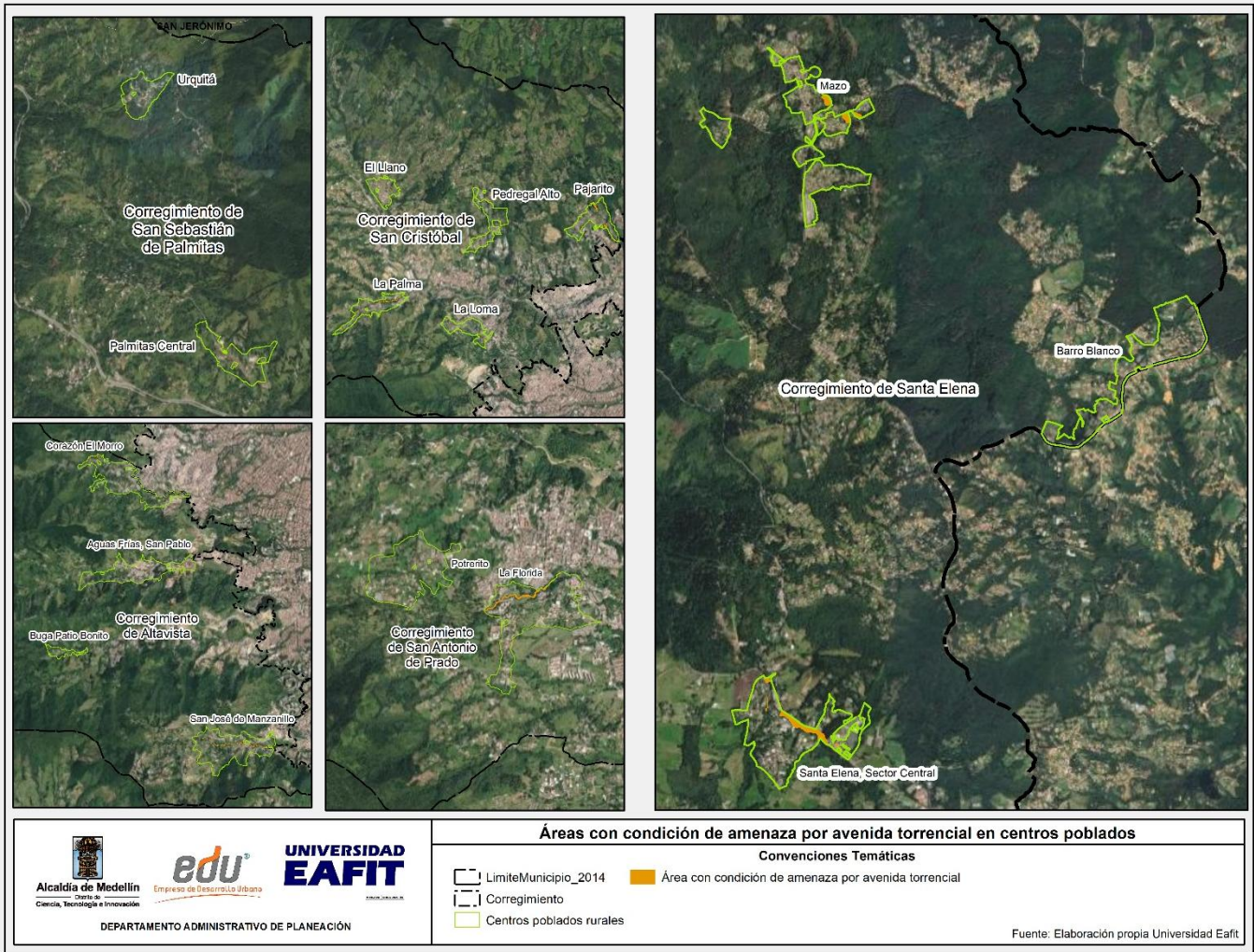
Ilustración 258. Áreas con condición de amenaza por avenidas torrenciales en centros poblados del Distrito de Medellín
