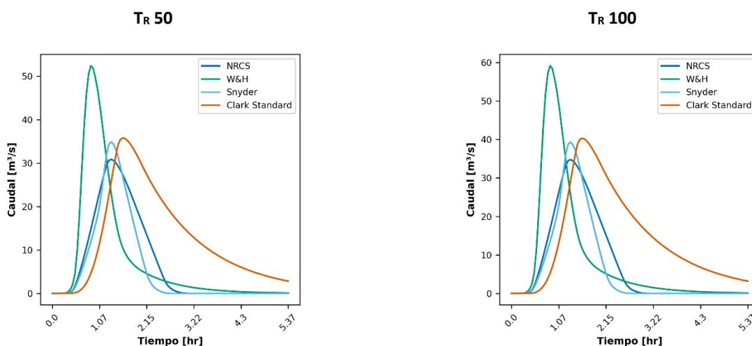
Ilustración 163. Hidrógrafa de respuesta de la quebrada Doña María para Tr 50 años (izquierda) y 100 años (derecha).
