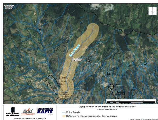
Ilustración 187. Fuentes hídricas incluidas en el modelo hidráulico La Puerta
