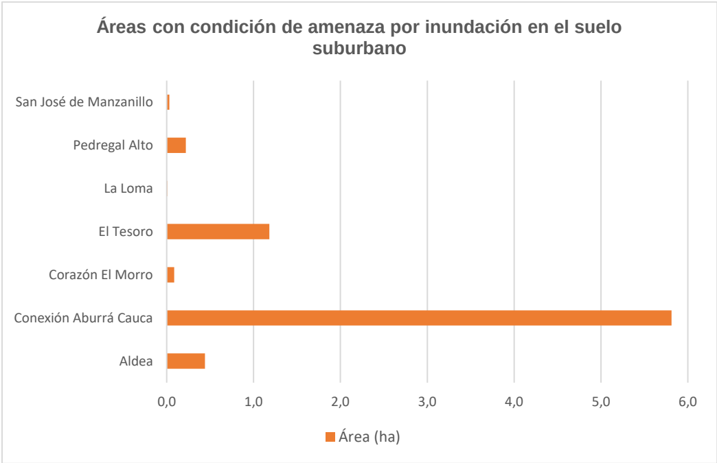
Ilustración 252. Áreas con condición de amenaza por inundaciones del suelo suburbano del Distrito de Medellín
