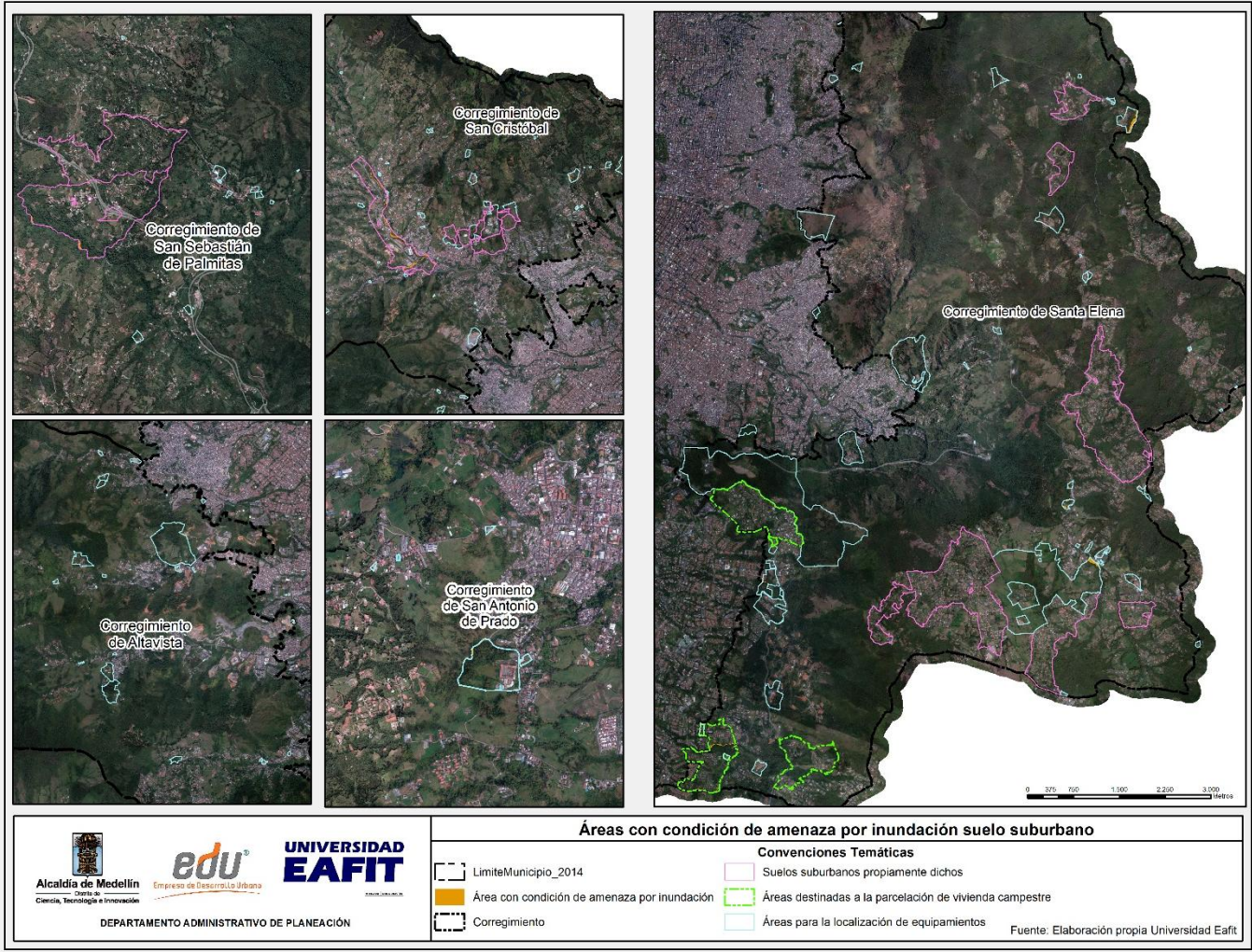
Ilustración 248. Áreas con condición de amenaza por inundación del suelo suburbano del Distrito de Medellín
