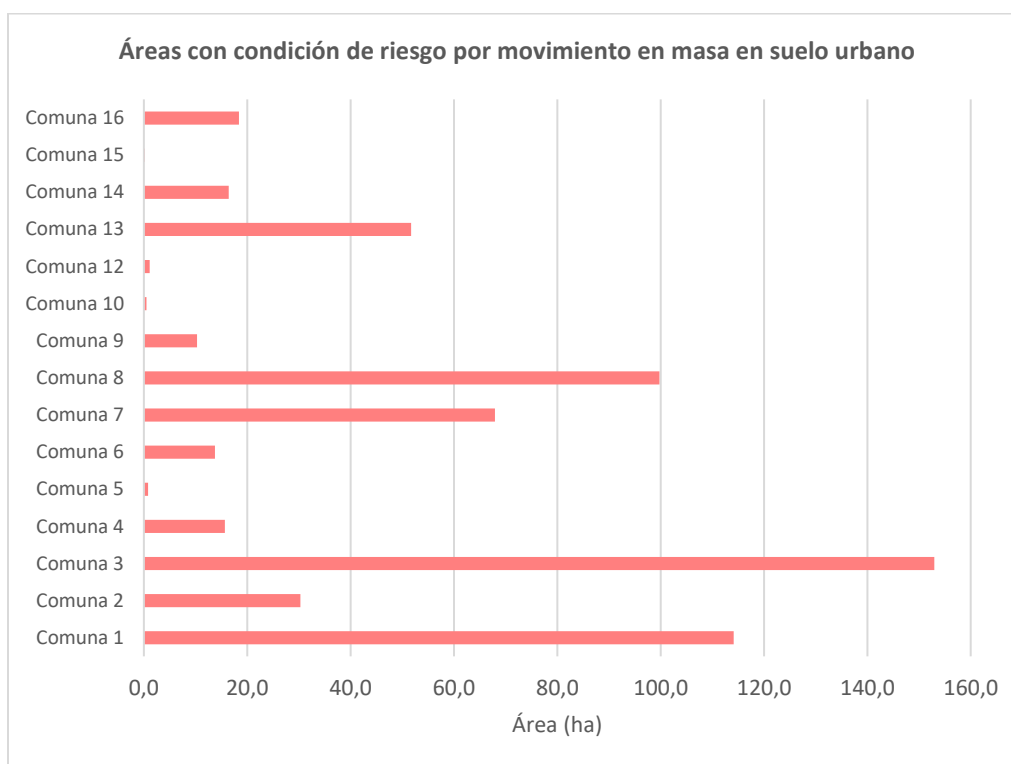
Ilustración 315. Áreas con condición de riesgo por polígono del suelo urbano del Distrito de Medellín
