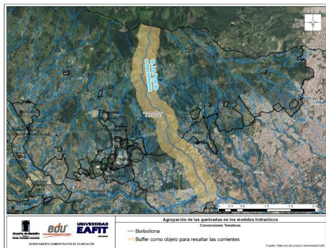
Ilustración 188. Fuentes hídricas incluidas en el modelo hidráulico La Borbollona
