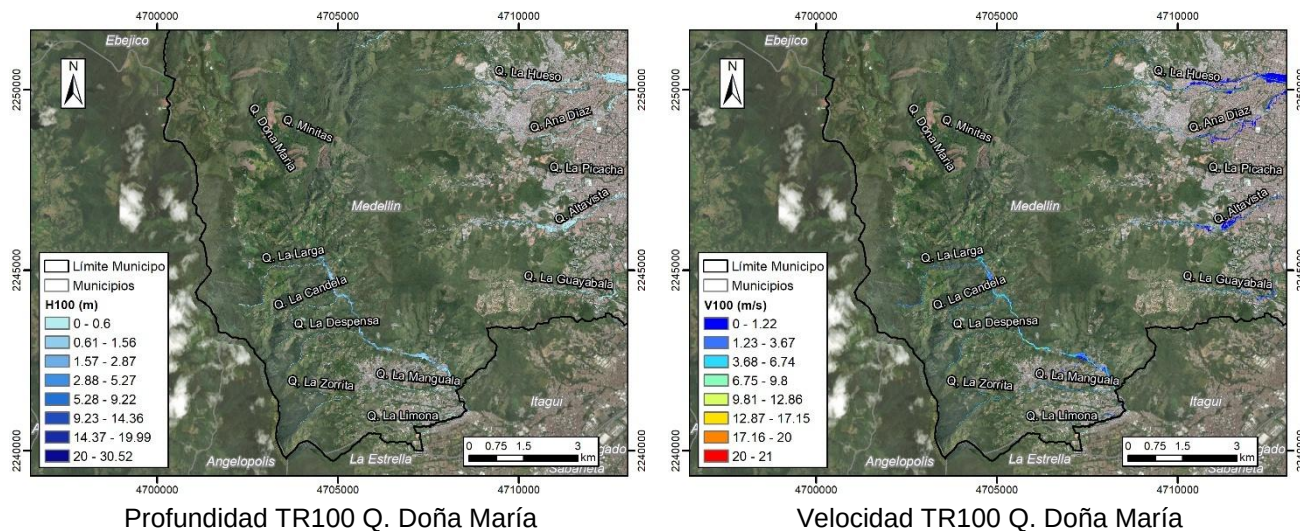
Ilustración 211. Campo de profundidad y velocidad para TR100 en quebrada Doña María
