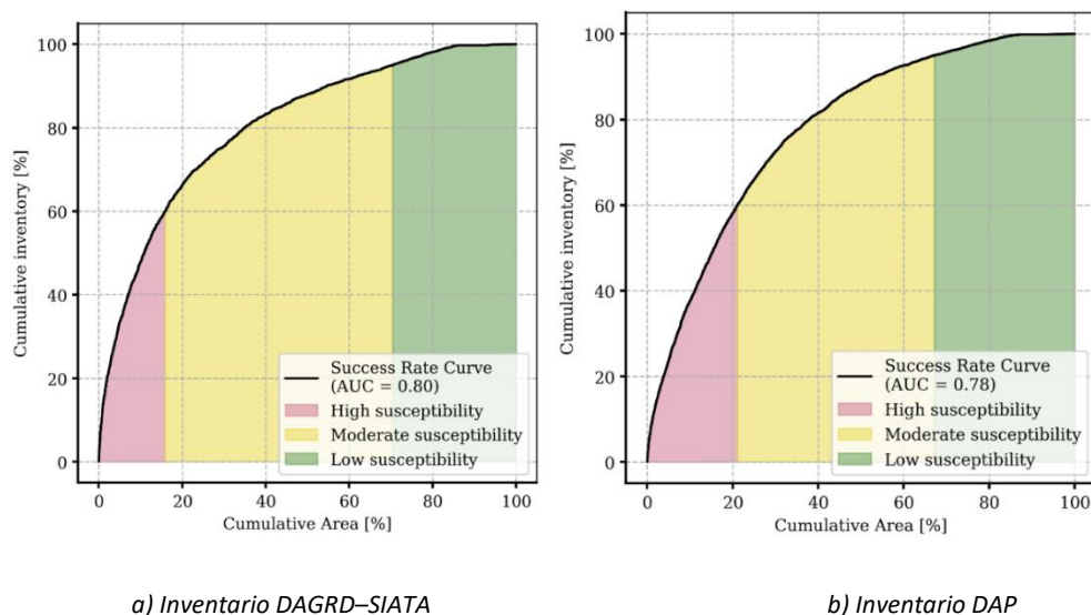
Ilustración 100. Curva de éxito, área bajo la curva y delimitación de umbrales para la zonificación por UL
