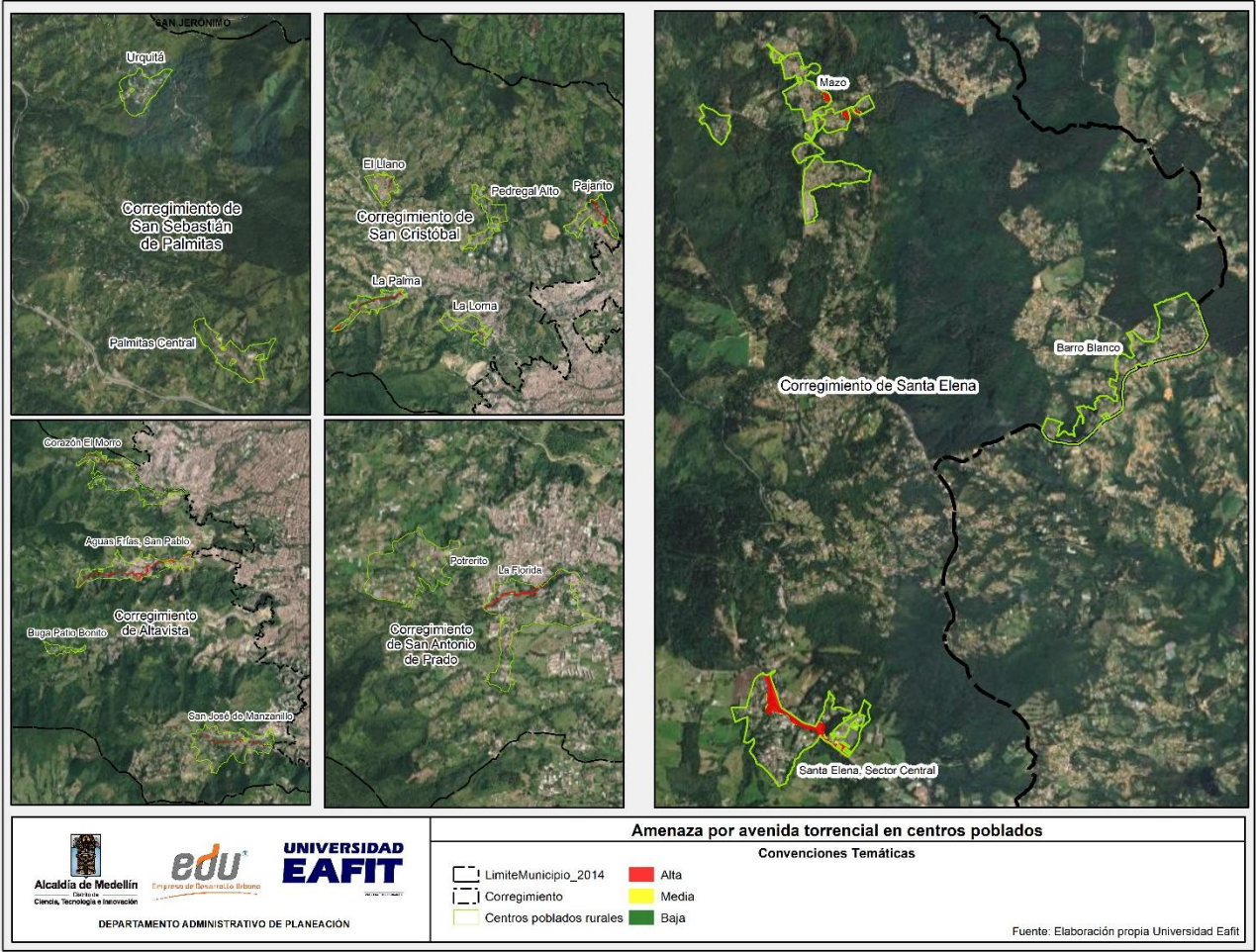
Ilustración 234. Amenaza por avenida torrencial en centros poblados del Distrito de Medellín
