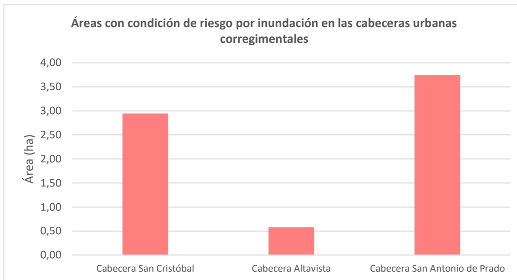
Ilustración 277. Áreas con condición de riesgo (ACR) por inundaciones de las cabeceras corregimentales del Distrito de Medellín
