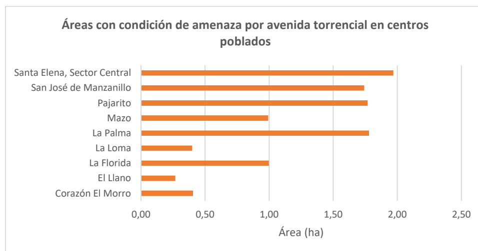
Ilustración 262. Áreas con condición de amenaza por avenidas torrenciales en los centros poblados del Distrito de Medellín
