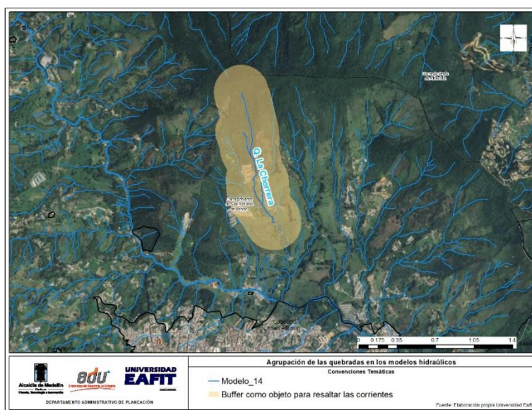
Ilustración 183. Fuentes hídricas incluidas en el modelo hidráulico 14
