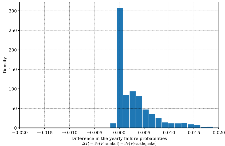
Ilustración 116. Diferencias en las probabilidades de falla anualizadas para los dos detonantes
