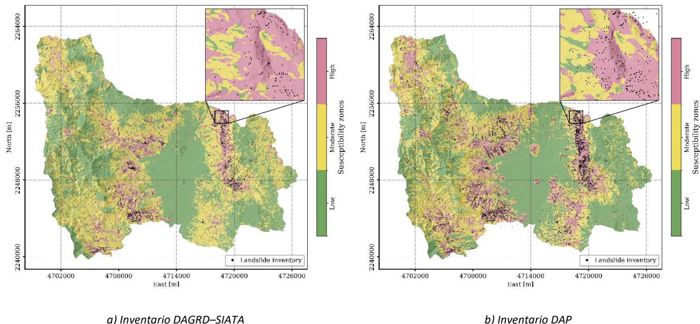
Ilustración 107. Zonificación de susceptibilidad por movimientos en masa a partir de UL en el Distrito de Medellín
