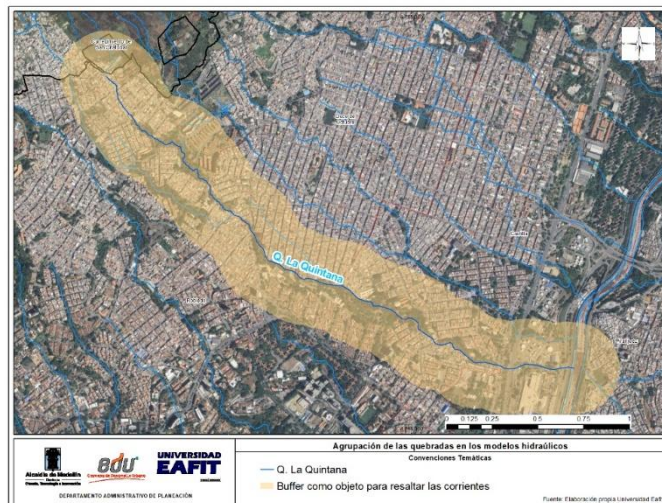
Ilustración 195. Fuentes hídricas incluidas en el modelo hidráulico La Quintana
