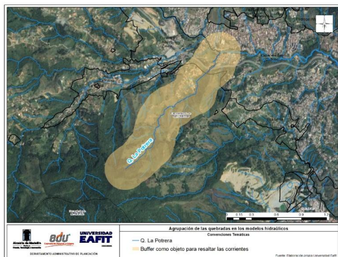
Ilustración 186. Fuentes hídricas incluidas en el modelo hidráulico La Potrera
