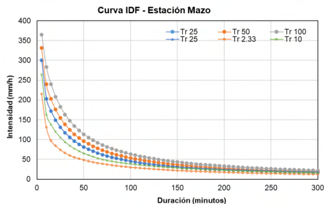
Ilustración 151. Curvas IDF para las estaciones Chorrillos y Mazo
