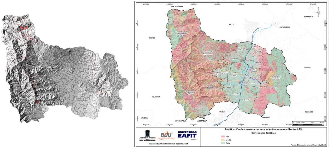
Ilustración 135. Áreas afectadas y zonificación de amenaza por índice de Probabilidad de Exposición a Propagación mayor a 25%.
