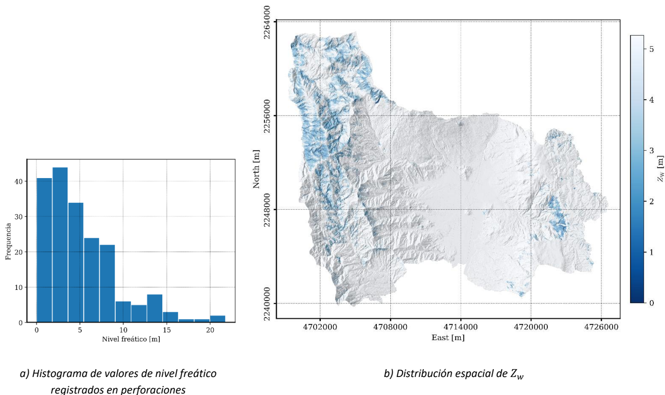
Ilustración 109. Distribución espacial de Z_w implementado en el Distrito de Medellín
