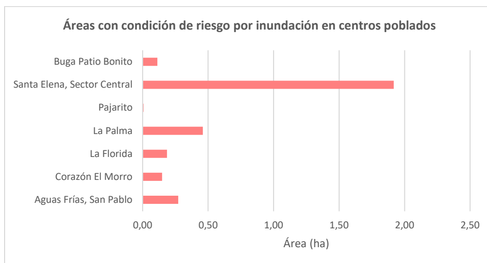
Ilustración 261. Áreas con condición de riesgo por inundaciones en los centros poblados del Distrito de Medellín
