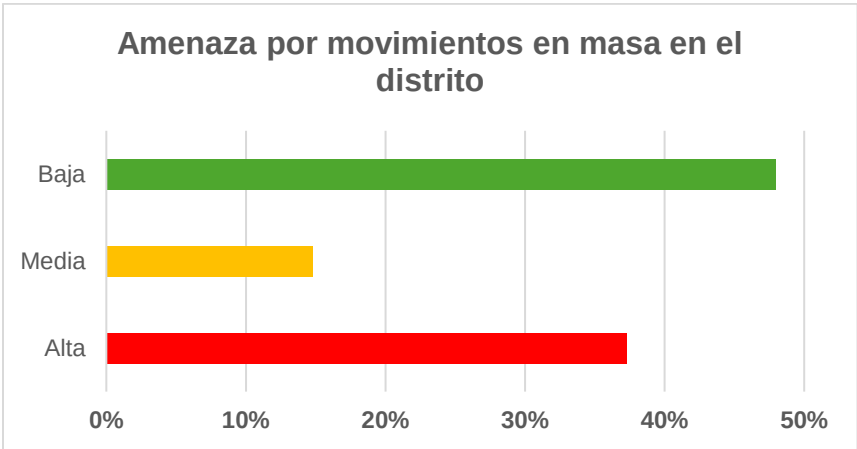
Ilustración 290. Distribución de la amenaza por movimientos en masa del Distrito de Medellín
