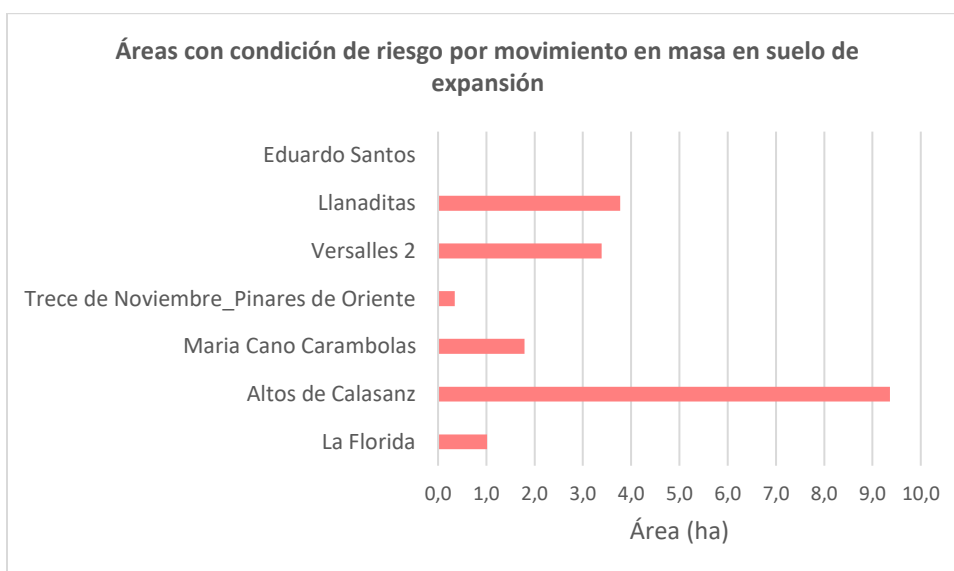
Ilustración 323. Áreas con condición de riesgo por polígono de los suelos de expansión del Distrito de Medellín
