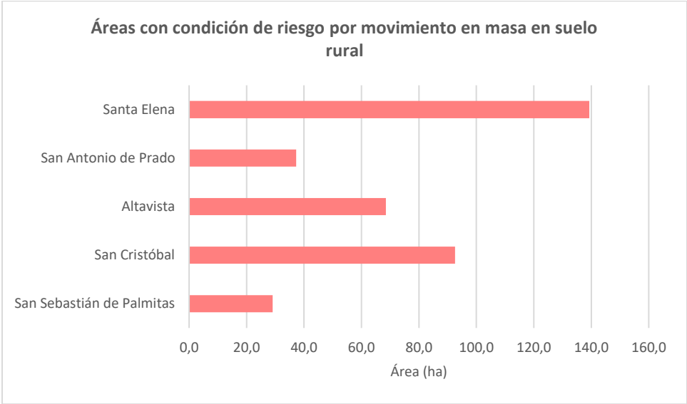
Ilustración 303. Distribución de las áreas con condición de riesgo del suelo rural del Distrito de Medellín
