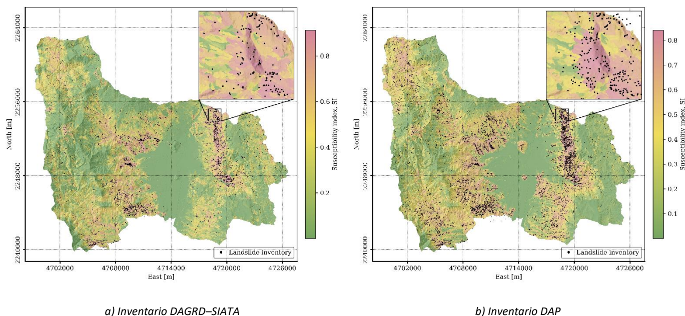
Ilustración 104. Índice de susceptibilidad por movimientos en masa a partir de UL en el Distrito de Medellín
