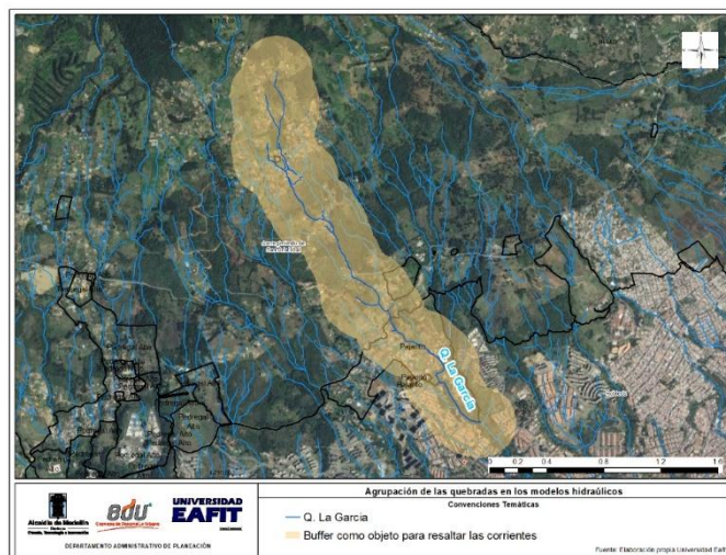
Ilustración 197. Fuentes hídricas incluidas en el modelo hidráulico La García
