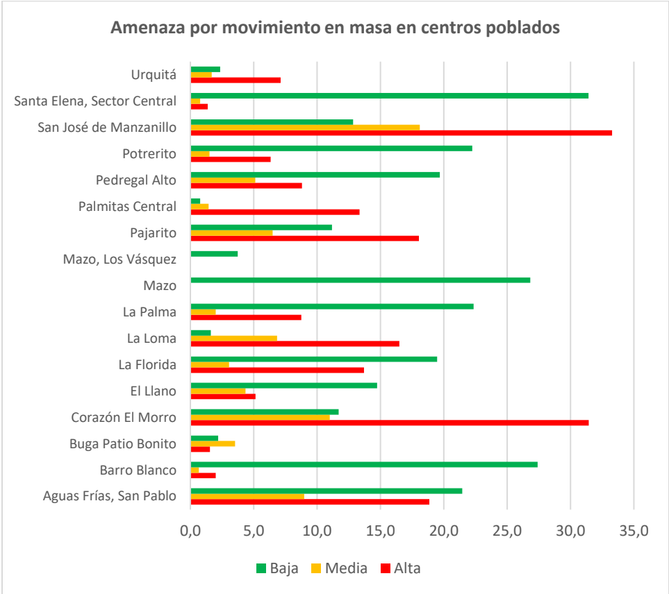
Ilustración 297. Distribución de amenaza por movimientos en masa por cada uno de los centros poblados del Distrito Fuente: Universidad EAFIT, 2025.
