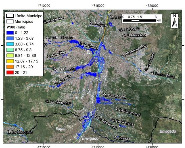
Velocidad TR100 Q. Santa Elena
