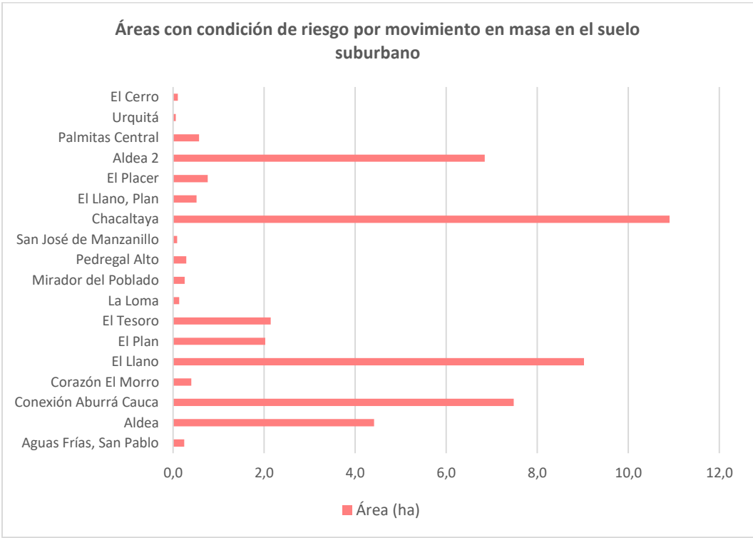
Ilustración 307. Áreas con condición de riesgo por polígono del suelo suburbano del Distrito de Medellín
