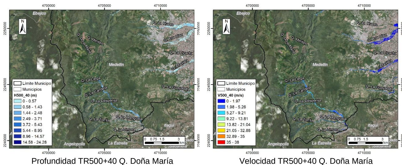
Ilustración 212. Campo de profundidad y velocidad para TR500+40 en quebrada Doña María
