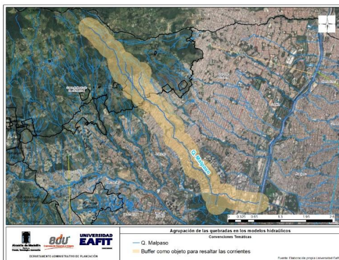
Ilustración 191. Fuentes hídricas incluidas en el modelo hidráulico La Malpaso
