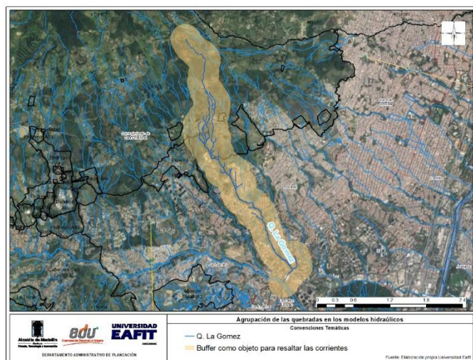
Ilustración 190. Fuentes hídricas incluidas en el modelo hidráulico La Gómez
