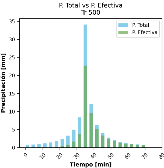
Ilustración 160. Aguacero de diseño en la quebrada La Presidenta
