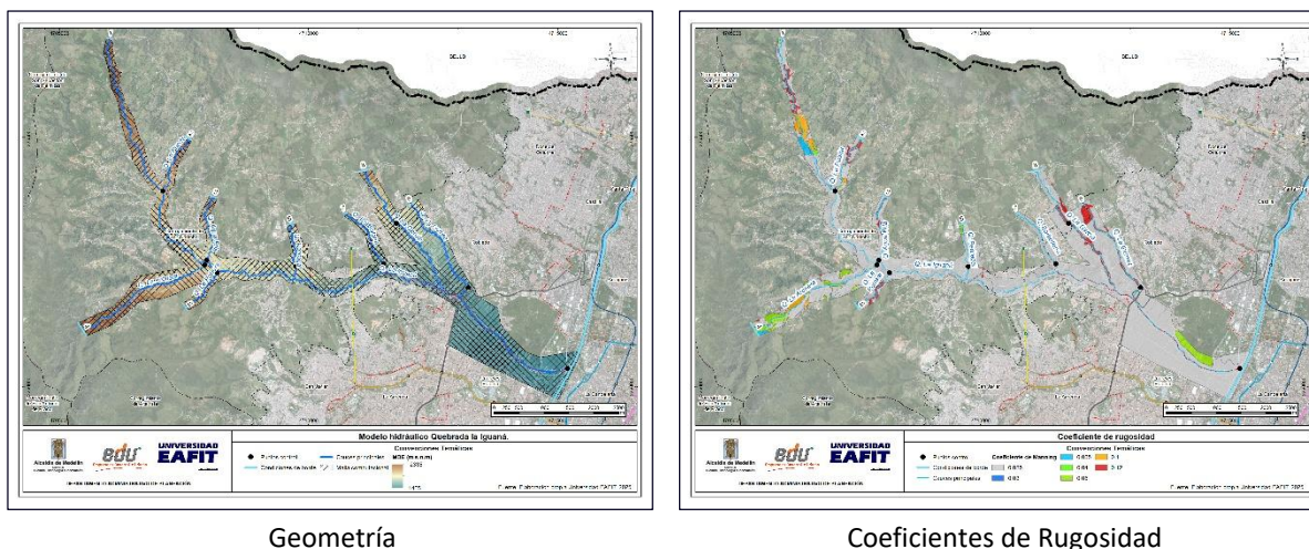
Ilustración 199. Modelo Hidráulico Bidimensional implementado para la Quebrada La Iguaña
