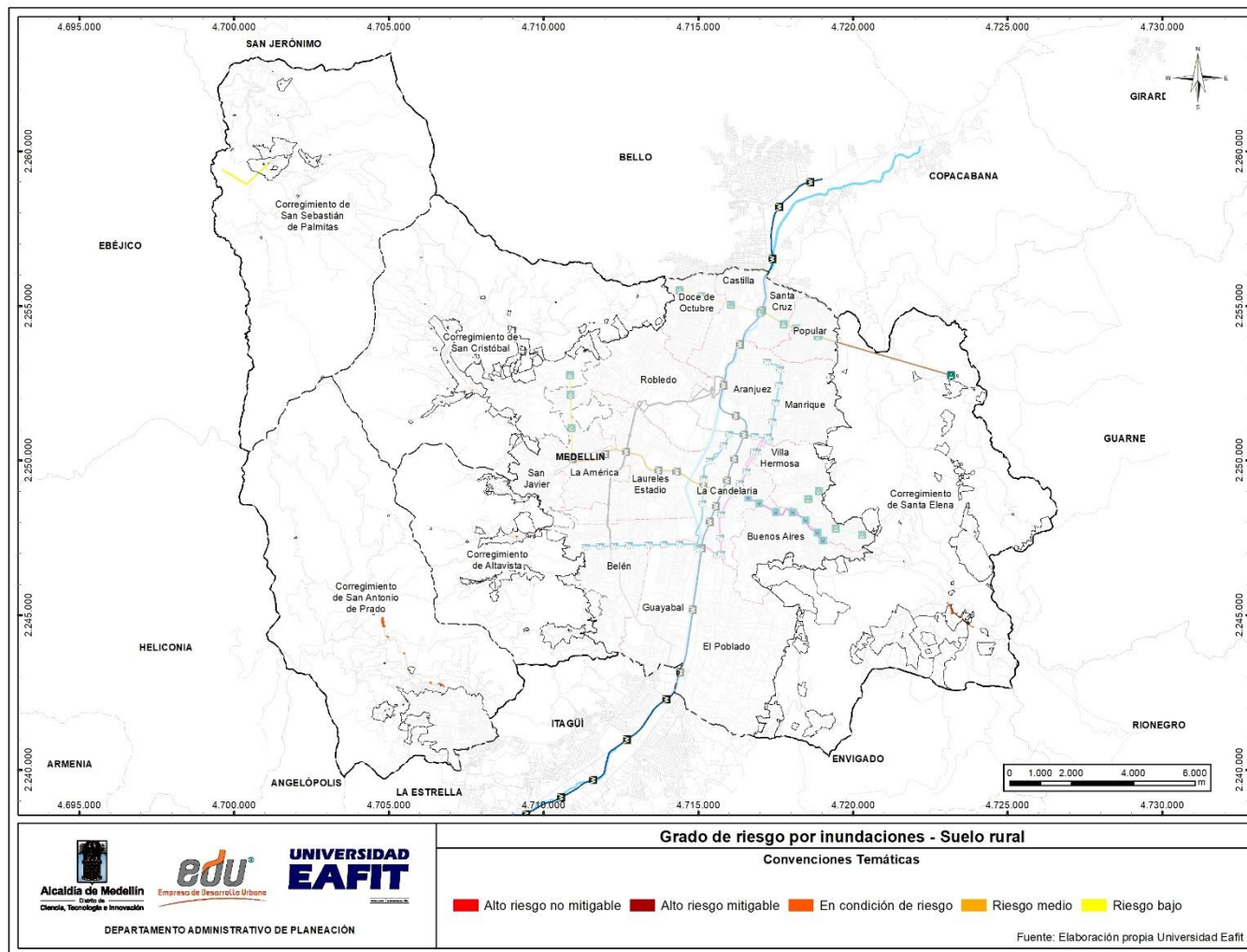
Ilustración 285. Áreas en la categoría de riesgo por inundación en estudios de detalle en el suelo rural
