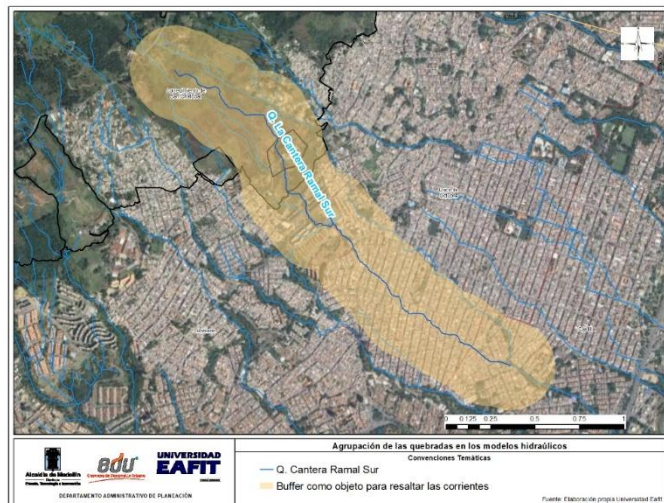
Ilustración 194. Fuentes hídricas incluidas en el modelo hidráulico La Cantera
