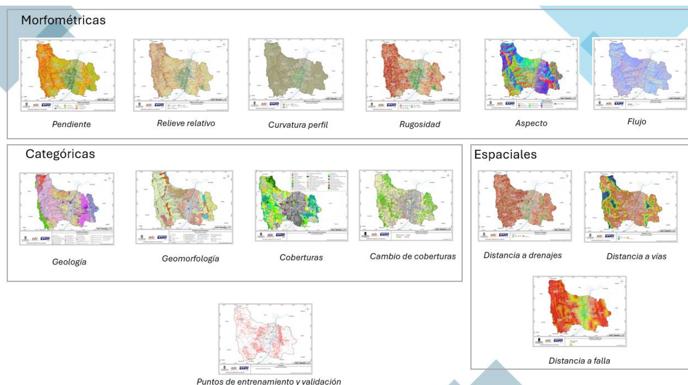
Ilustración 87. Variables utilizadas en el modelo
