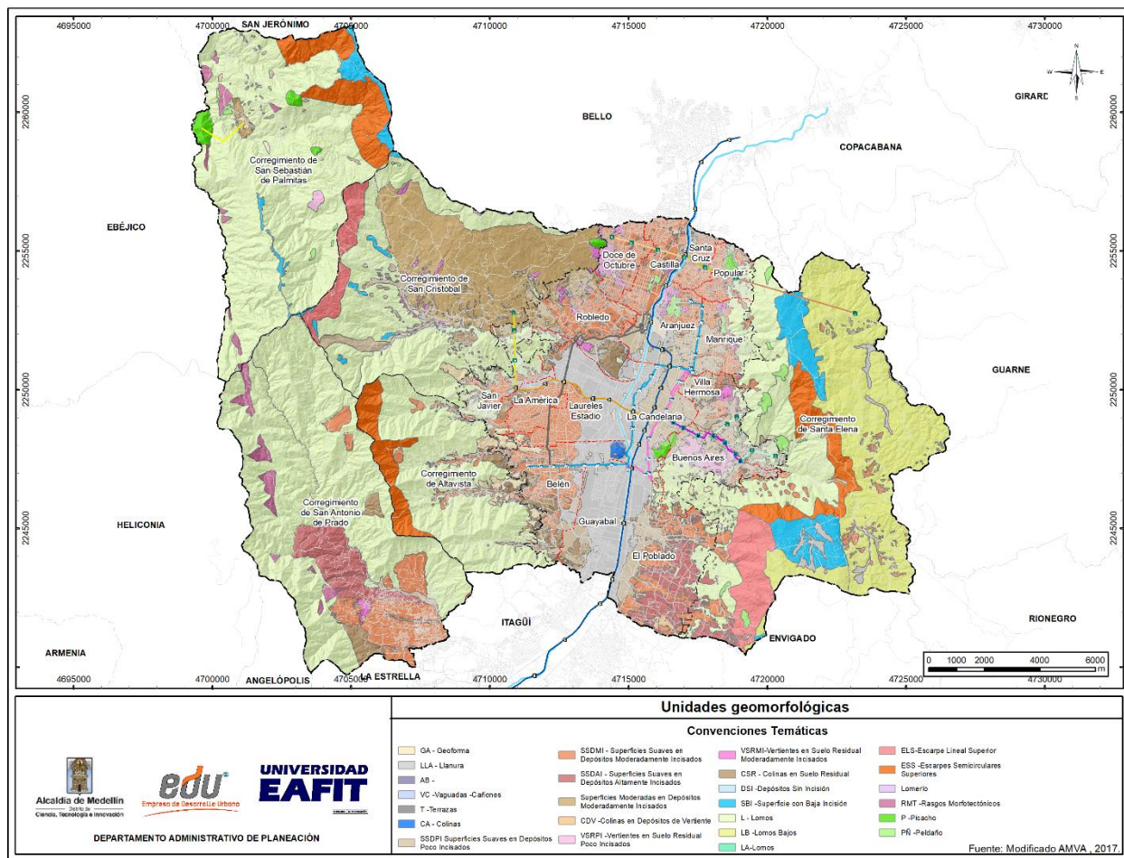
Ilustración 26. Mapa de unidades geomorfológicas del Distrito de Medellín
