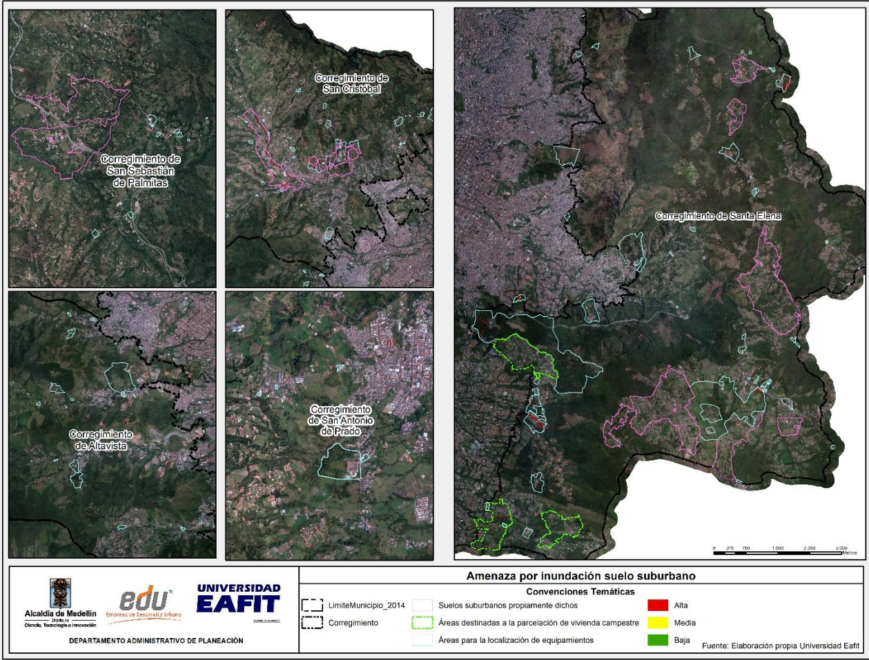
Ilustración 220. Amenaza por inundación del suelo suburbano del Distrito de Medellín
