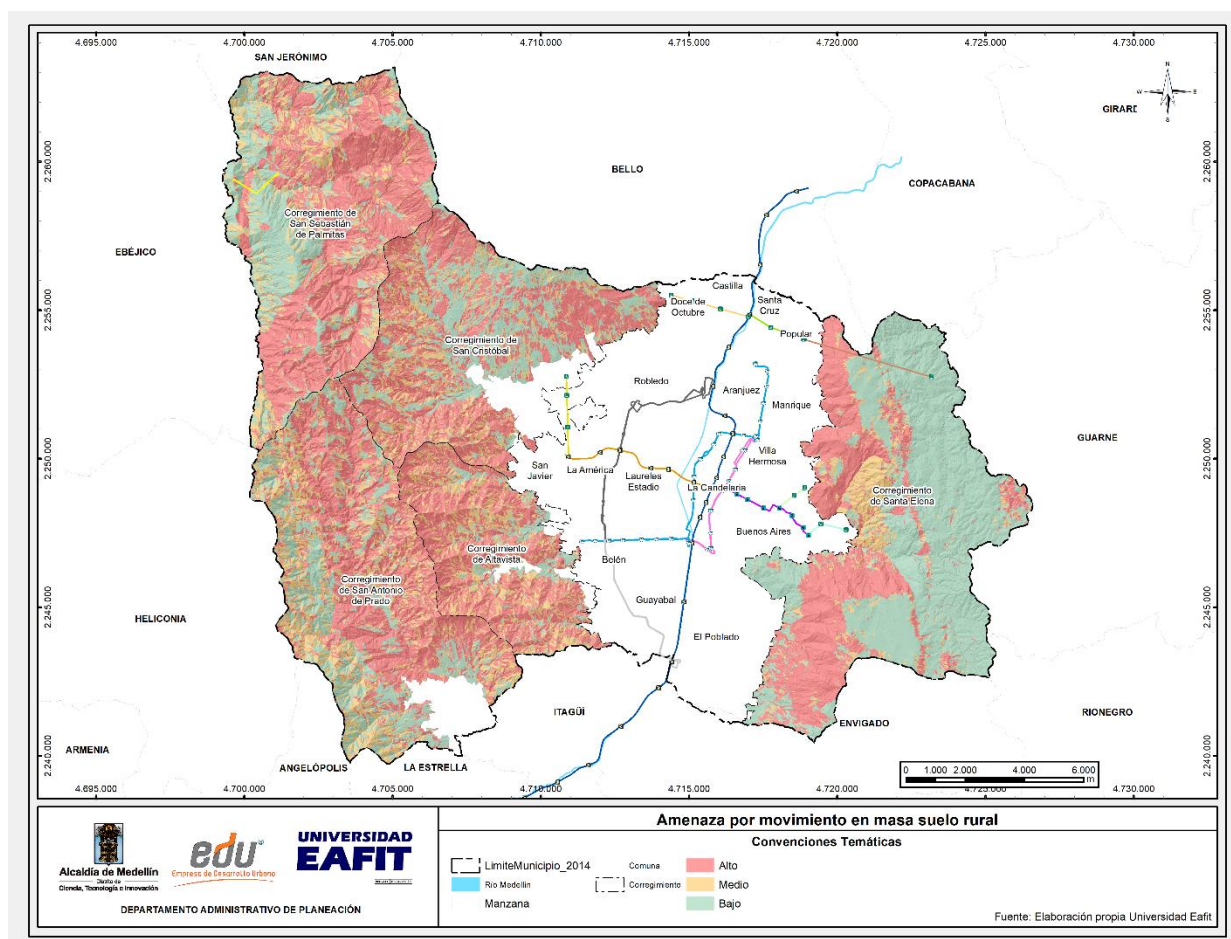
Ilustración 292. Amenaza por movimientos en masa del suelo rural del Distrito de Medellín
