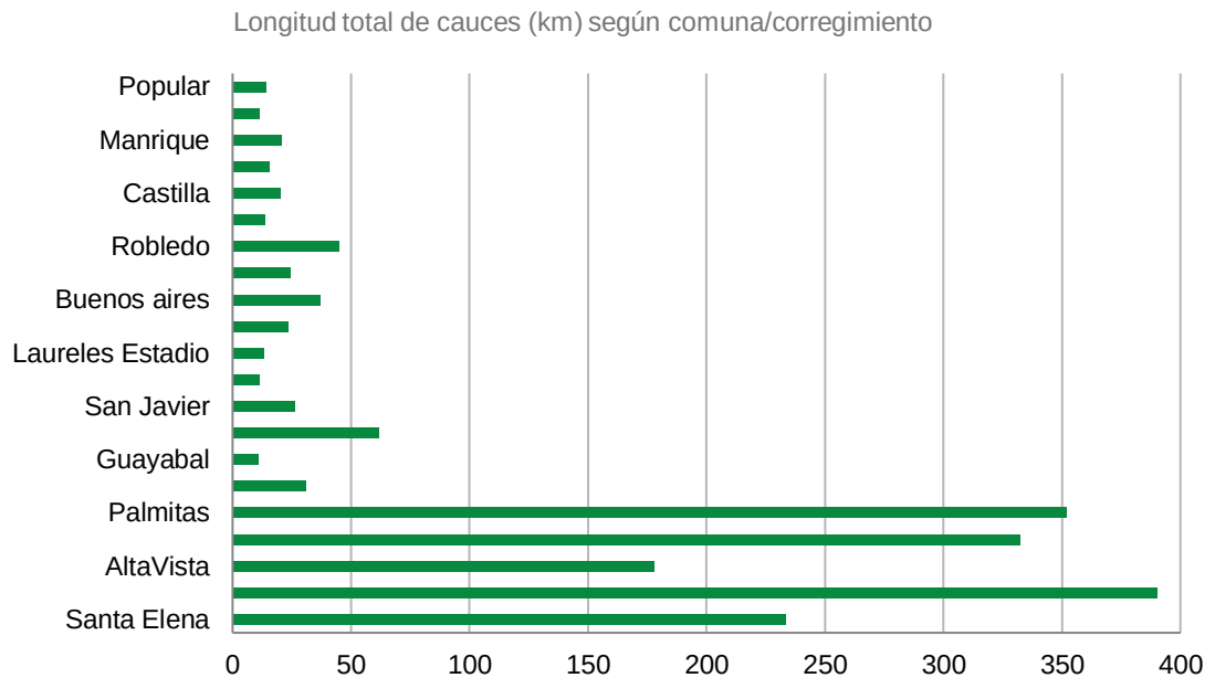
Gráfica 134: Recurso hídrico superficial en el distrito de Medellín.
