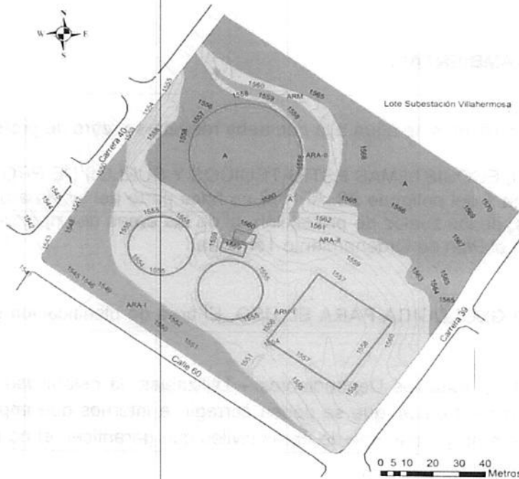
Plano N° 4. Zonificación geológica y geotécnica de la Zona 1 del polígono Z3_API_13.
