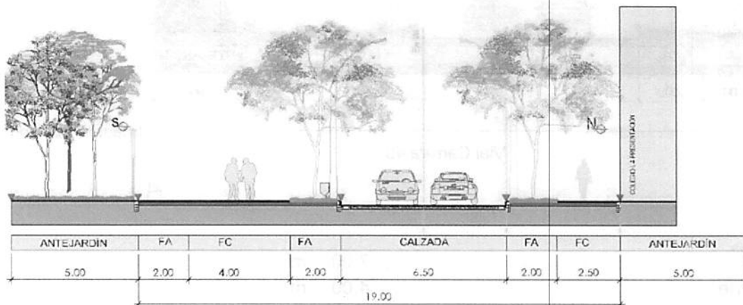
Sección Vial Calle 62 Urabá.
